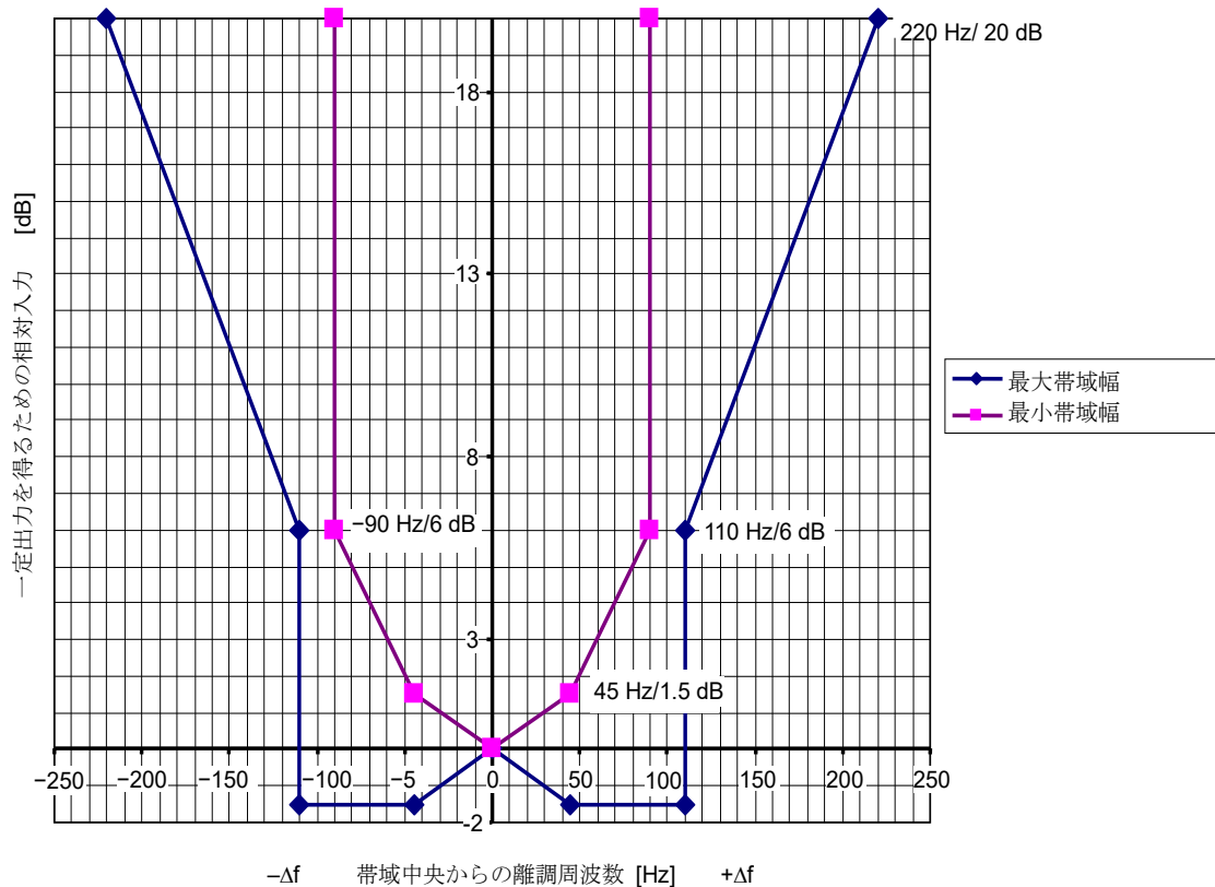
図 1 - 総合選択度の許容範囲ー通過帯域 (バンド A)
