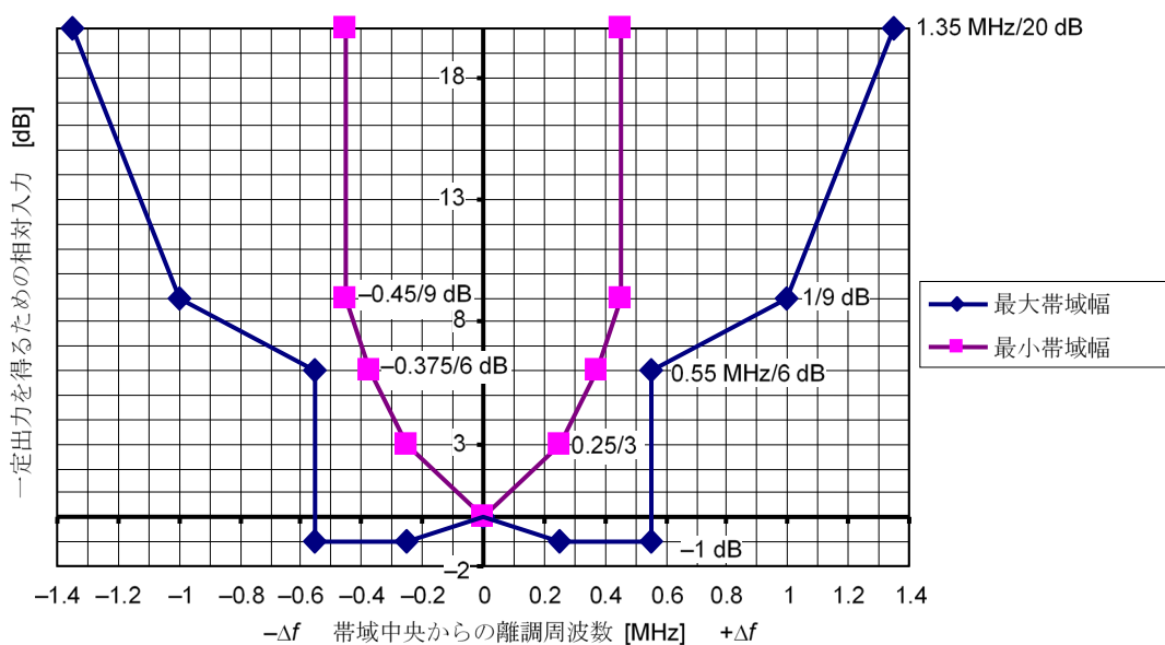
図 3 - 総合選択度の許容範囲－通過帯域（バンド C 及び D）
