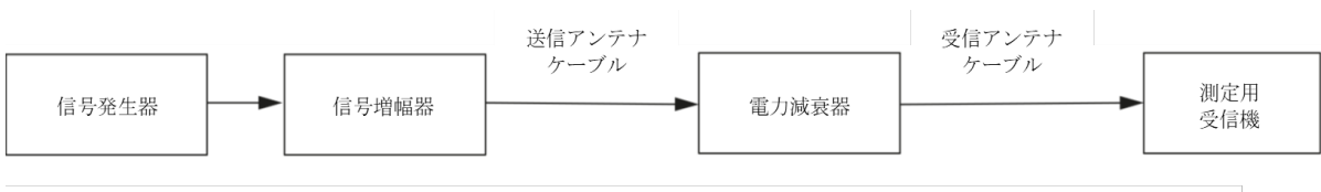
図 38 - 電力増幅器と減衰器を用いた V_{\text{DIRECT}} の測定構成
