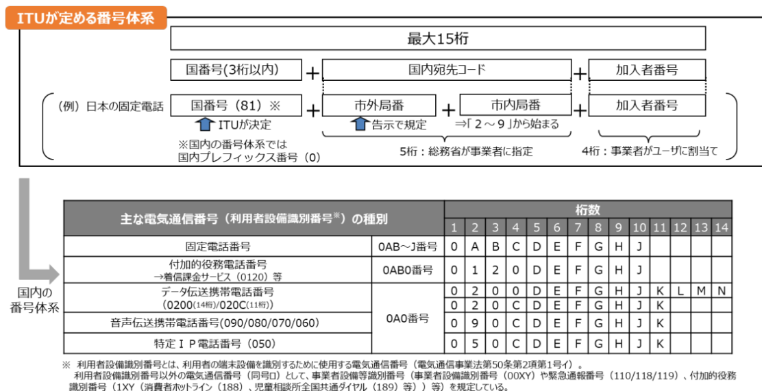
図 10 電気通信番号の体系
