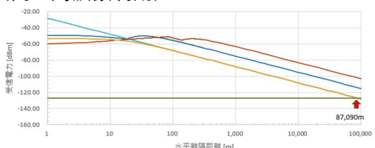
参照図-2-8 RKE E.I.R.P.: 0dBm
