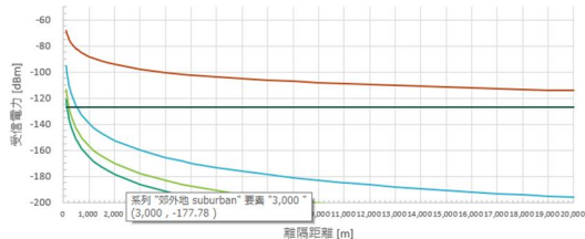
参照2-22 RKE E.I.R.P.: 0dBm
