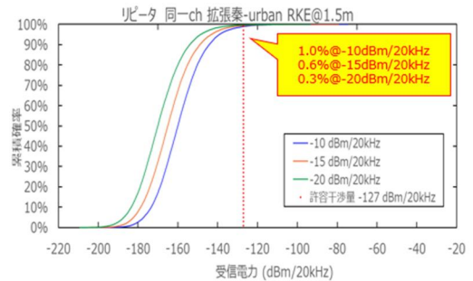
参图 4-26 RKE からアマチュア局（移動・車載/ハンディ（左）、固定・レピータ（ホイップ）（右））への干渉発生確率（同一帯域利用、普及予測パターン 1）
