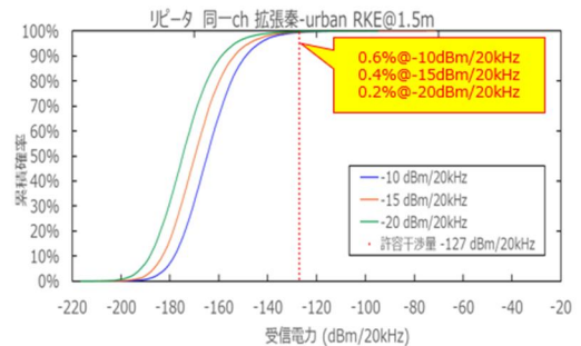
参图 4-27 RKE からアマチュア局（移動・車載/ハンディ（左）、固定・レピータ（ホイップ）（右））への干渉発生確率（同一帯域利用、普及予測パターン 2）
