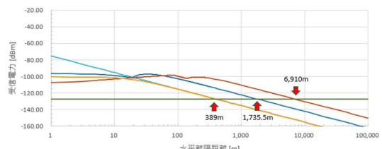
参照図-2-6 TPMS帯域外 -36.02dBm/100kHz (-43.01dBm/20kHz)
