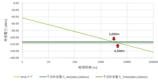
参考図2-33 自由空間損失のみ
