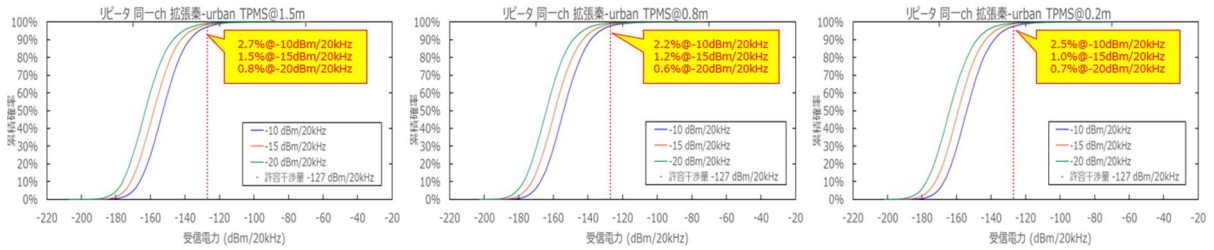
参图 4-10 TPMS からアマチュア局（固定・レピータ（ホイップ））への干渉発生確率（同一帯域利用、普及予測パターン 1）
