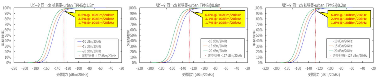
参图 4-12 TPMS からアマチュア局（固定・レピータ（コリニアアンテナ））への干渉発生確率（同一帯域利用、普及予測パターン 1）
