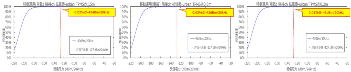
参图 4-18 TPMS からアマチュア局（移動・車載/ハンディ）への干渉発生確率 （隣接帯域利用、普及予測パターン 1）
