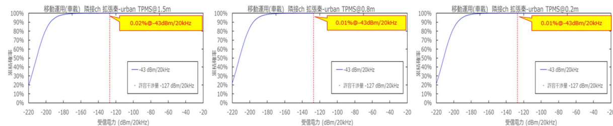
参图 4-19 TPMS からアマチュア局（移動・車載/ハンディ）への干渉発生確率 （隣接帯域利用、普及予測パターン 2）
