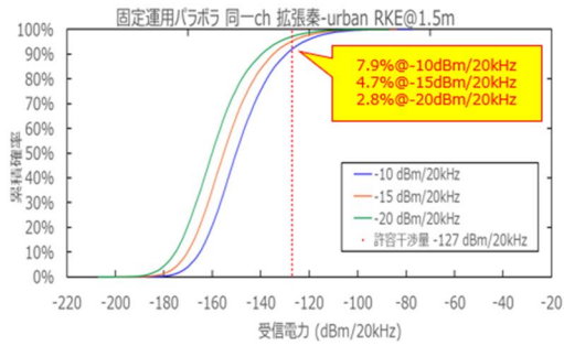
参图 4-25 RKE からアマチュア局（固定・パラボラ（左）、固定・八木（右））への干渉発生確率（同一帯域利用、普及予測パターン 2）
