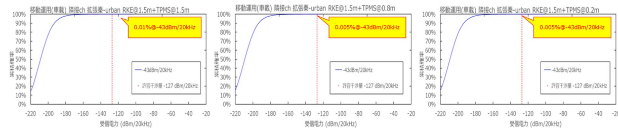
参図 4-49 TPMS 及び RKE からアマチュア局（移動・車載/ハンディ）への干渉発生確率（隣接帯域利用、普及予測パターン 2）
