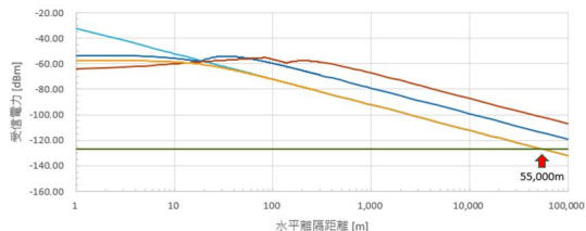
参照図-2-4 TPMS E.I.R.P.: 0dBm
