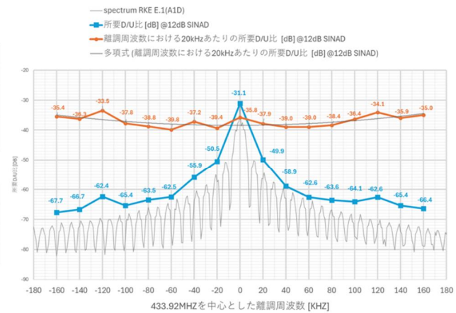
参図 5-3 干渉波:433.92MHz±160kHz で所要 D/U 比を測定した結果 (ASK (RKE2))
