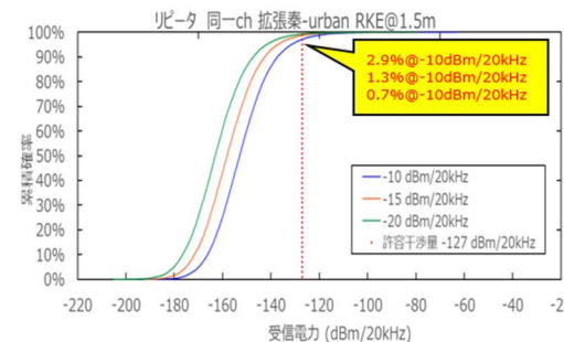
参图 4-28 RKE からアマチュア局（固定・レピータ（コリニアアンテナ））への干渉発生確率（同一帯域利用、普及予測パターン 1（左）、普及予測パターン 2（右））
