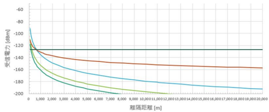
参照2-21 RKE 帯域外 -36.02dBm/100kHz (-43.01dBm/20kHz)
