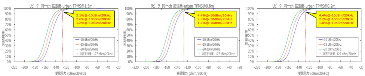
参图 4-13 TPMS からアマチュア局（固定・レピータ（コリニアアンテナ））への干渉発生確率（同一帯域利用、普及予測パターン 2）
