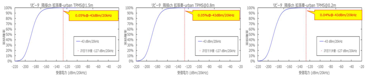
参图 4-21 TPMS からアマチュア局（固定・レピータ（ホイップ））への干渉発生確率 （隣接帯域利用、普及予測パターン 2）
