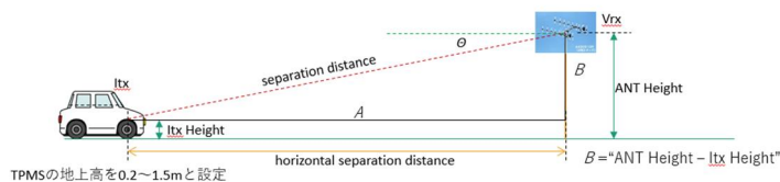
参照図-2-7 シミュレーションモデル
