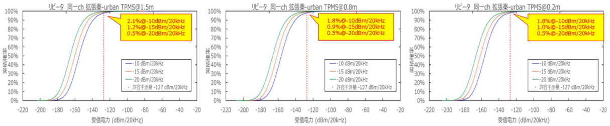
参图 4-11 TPMS からアマチュア局（固定・レピータ（ホイップ））への干渉発生確率（同一帯域利用、普及予測パターン 2）
