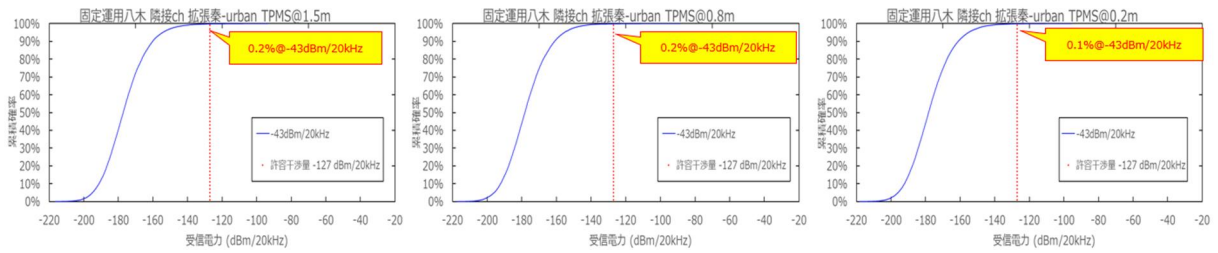
参图 4-17 TPMS からアマチュア局（固定・八木）への干渉発生確率 （隣接帯域利用、普及予測パターン 2）
