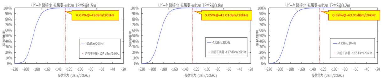
参图 4-20 TPMS からアマチュア局（固定・レピータ（ホイップ））への干渉発生確率 （隣接帯域利用、普及予測パターン 1）
