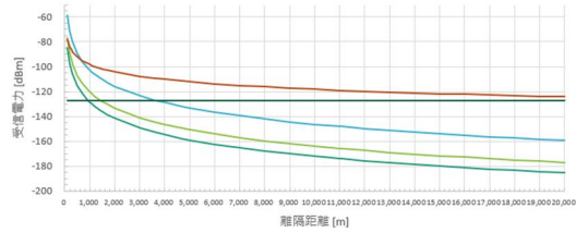
参照2-19 RKE E.I.R.P.: 0dBm
