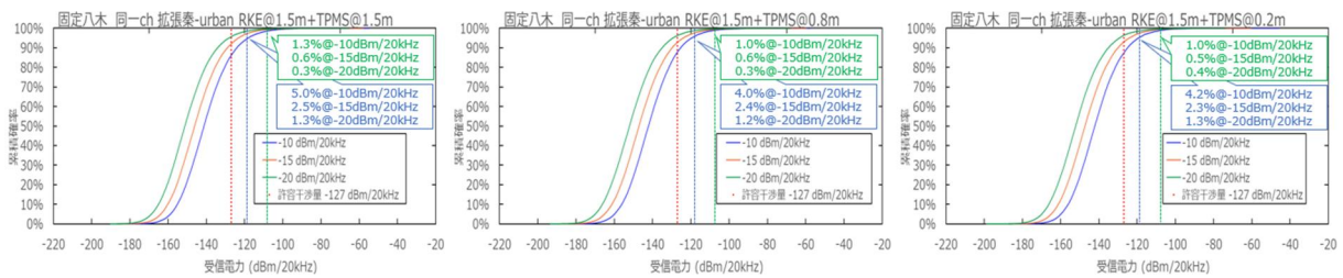
参図 4-56 実運用を想定した推定値に基づく TPMS 及び RKE からアマチュア局 (固定・八木) への干渉発生確率 (同一帯域利用、普及予測パターン 1)
