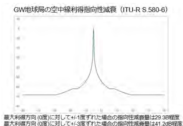
図 2. 1. 3. 2-2 GW 地球局の空中線利得指向性減衰
