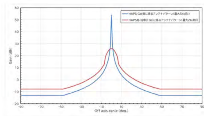
図2.3.9.1-1 HAPS局とHAPS GW局のアンテナパターン(アップリンク)
