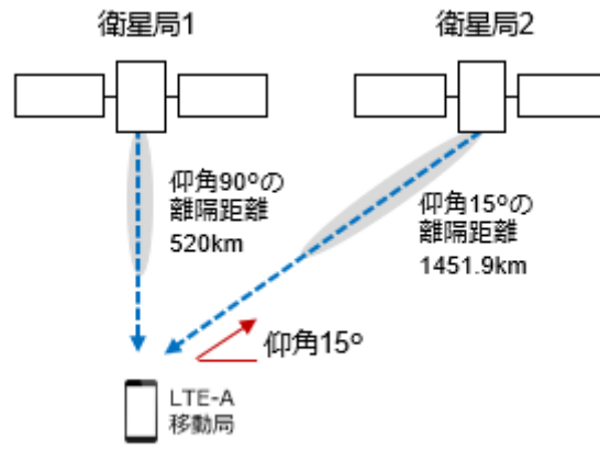
図 2. 2. 4. 2-1 700MHz 帯非静止衛星通信システム（衛星局）から LTE 移動通信システム（移動局）（隣接）への与干渉の対向モデル
