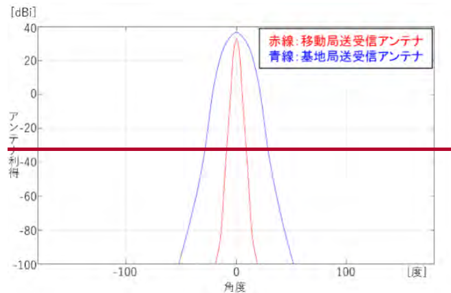
図2. 3. 10. 2-2 列車無線システム（基地局）の指向性減衰特性（垂直面）
