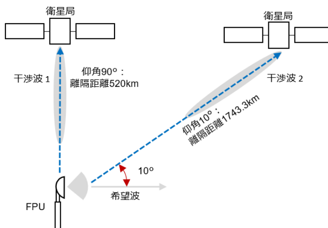
図 2. 3. 5. 4-2 FPU から 700MHz 帯非静止衛星通信システム (衛星局) への与干渉の実運用モデル
