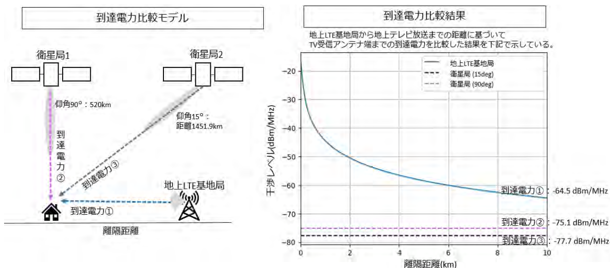
図2. 2. 2. 2-1 衛星局及び地上の移動通信システムLTE（基地局）からの一定離隔距離での到達電力の比較結果
