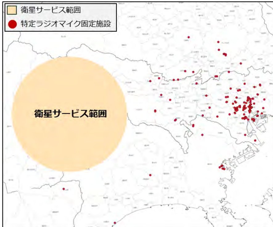
図 2. 2. 1. 3-3-4 特定ラジオマイク固定施設と衛星サービス範囲
