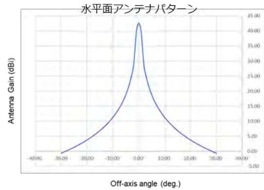
図 2. 3. 3. 5-4 一般業務用固定局の指向性減衰特性
