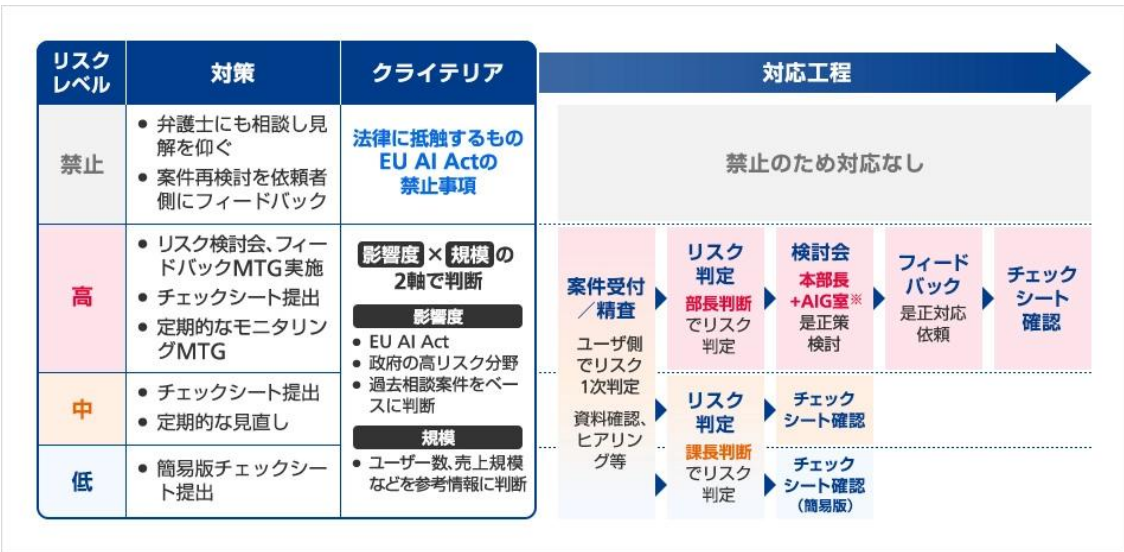
図 23.ソフトバンクのリスクベースアプローチ
