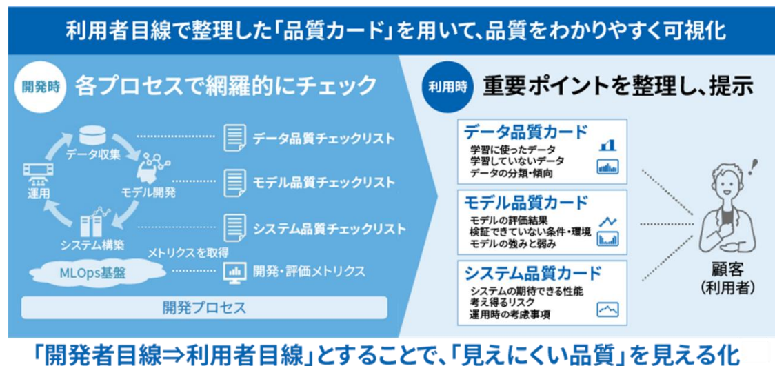
図 11. AI 品質保証ガイドライン・品質カード活用の流れ
