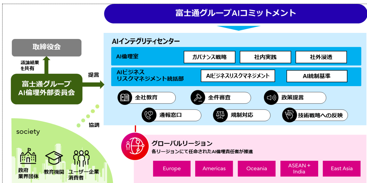
図 17. AI ガバナンスの体制
