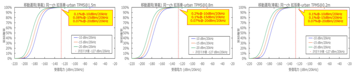
参图 4-8 TPMS からアマチュア局（移動・車載/ハンディ）への干渉発生確率 （同一帯域利用、普及予測パターン 1）
