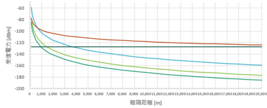
参照2-20 RKE E.I.R.P.: -10dBm
