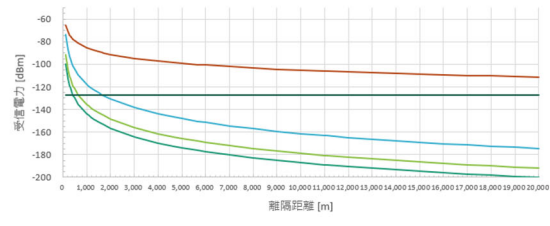
参图2-17 RKE E.I.R.P.: -10dBm
