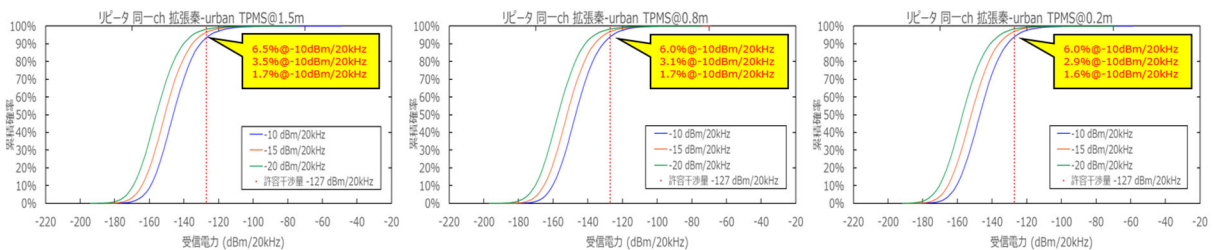
参图 4-12 TPMS からアマチュア局（固定・レピータ（コリニアアンテナ））への干渉発生確率（同一帯域利用、普及予測パターン 1）
