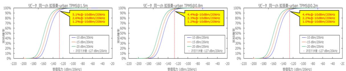
参图 4-13 TPMS からアマチュア局（固定・レピータ（コリニアアンテナ））への干渉発生確率（同一帯域利用、普及予測パターン 2）
