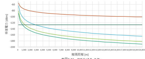
参图2-16 RKE E.I.R.P.: 0dBm
