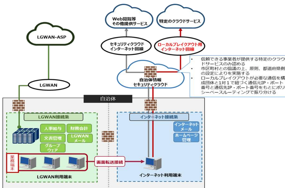
図表 35 ローカルブレイクアウト
