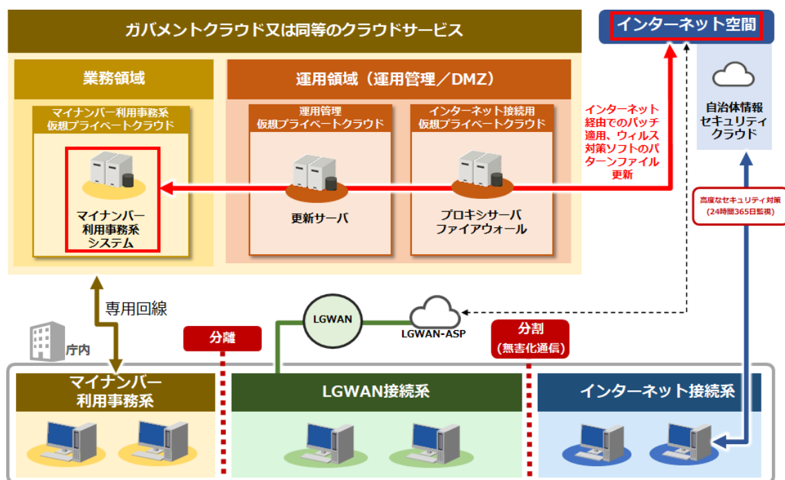
図表 55 インターネット経由による標準準拠システム等の修正プログラム適用、ウイルス対策ソフトのパターンファイル更新等のイメージ
