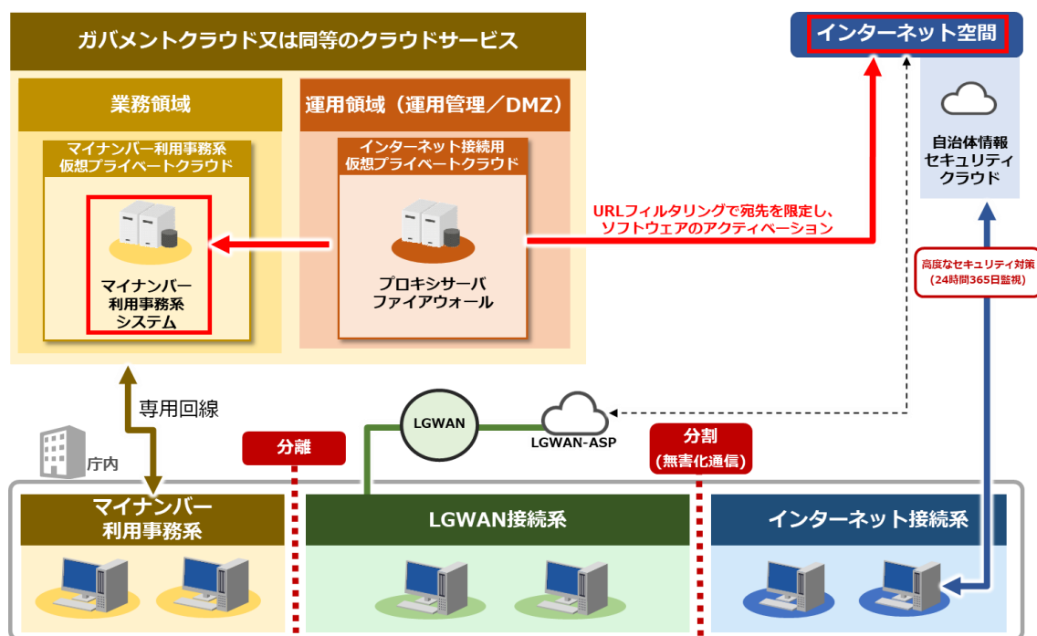
図表 56 インターネット経由での標準準拠システム等のソフトウェアの アクティベーションを実施する場合のイメージ
