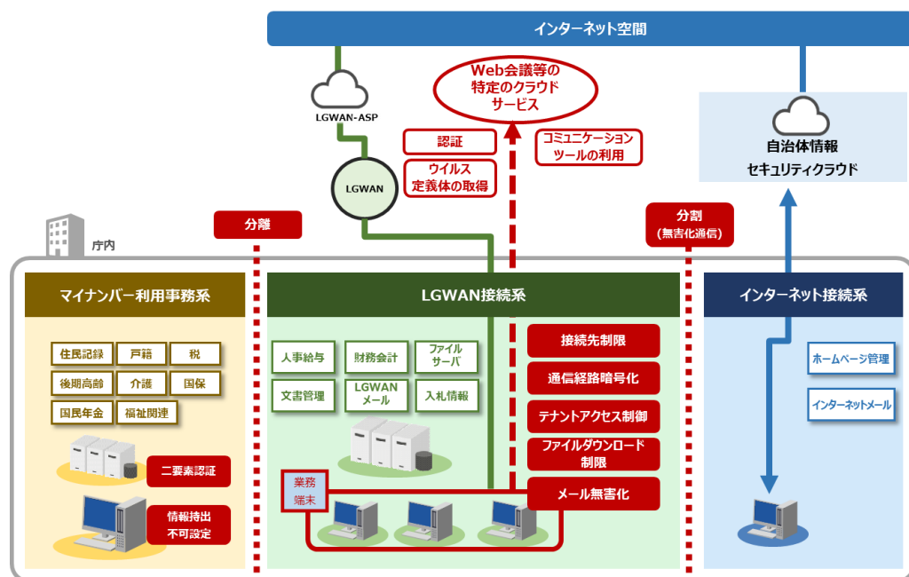
図表 31 αモデル（コミュニケーションツールを利用するが、ファイルを内部に取り込まない場合）イメージ図
