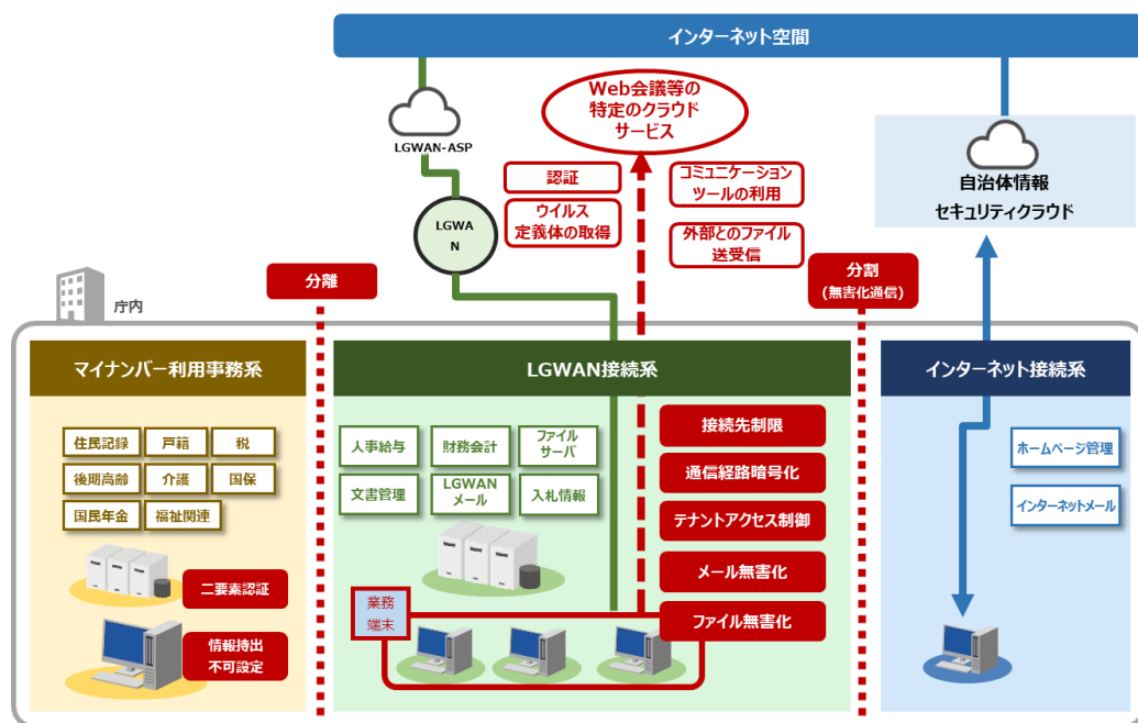
図表 33 α'モデル（コミュニケーションツールを利用し、外部とファイル送受信を行う場合）イメージ図
