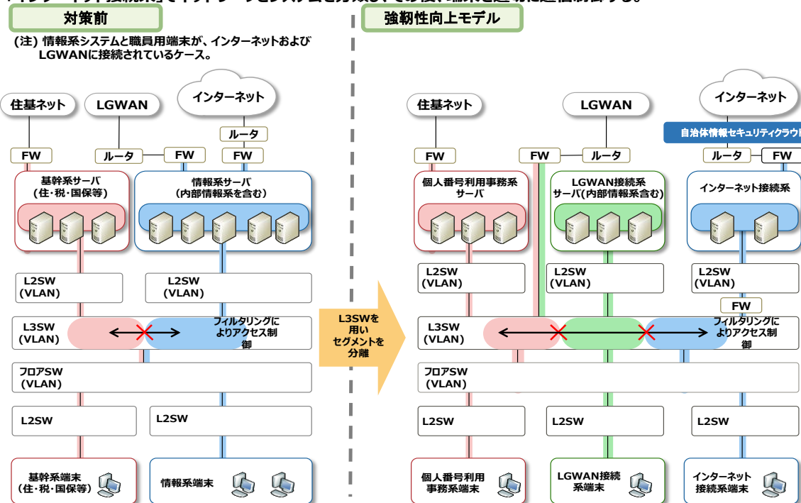
図表 25 強靱性向上モデルにおけるネットワーク再構成の一つのイメージ
