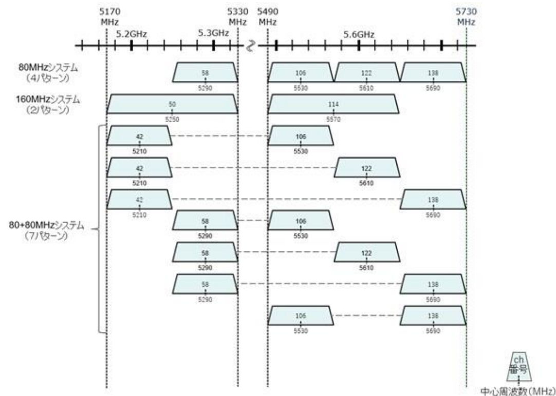
パンクチャリングが適用可能な5.2/5.3/5.6 GHz帯のチャネル配置
