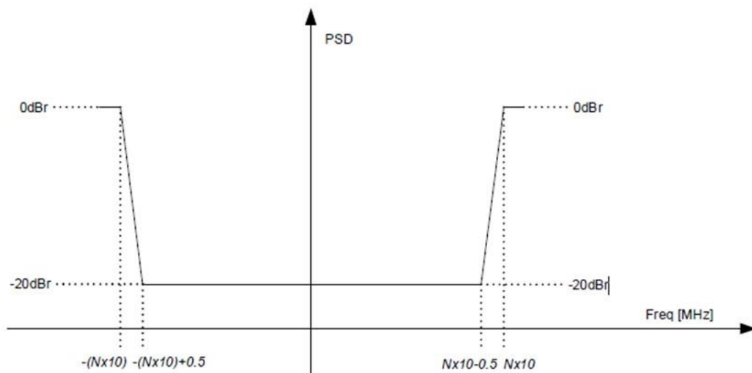
図 3-7 802.11ax で端以外の 20 MHz サブチャンネル×N 個をパルクチャしたスペクトラムマスクの例(参照 : IEEE Std 802.11ax-2021、Figure 27-52)
