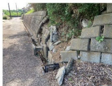
擁壁のハラミ ブロックの脱落
