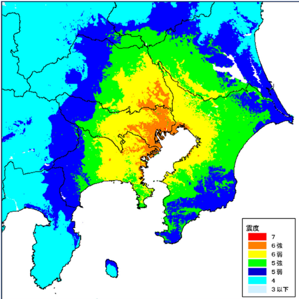
地震の規模：モーメントマグニチュード7.3
