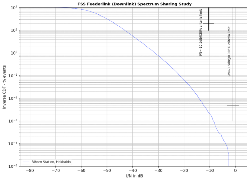
図 2-16 : アグリゲート干渉検討のシミュレーション結果
