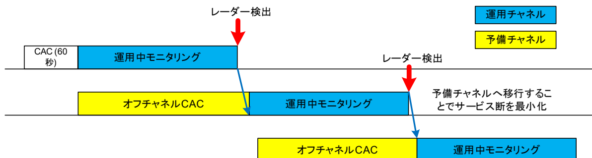
図 3-8 オフチャネル CAC の概念
