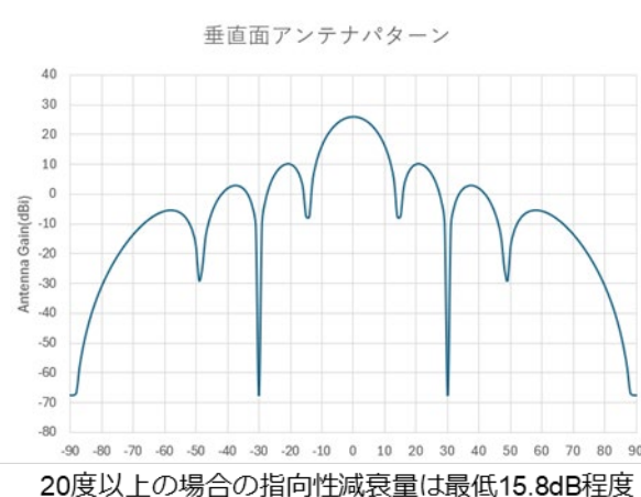
図 2. 3. 1. 2-3 5G 基地局の指向性減衰特性(垂直)
