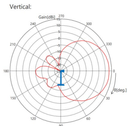
図2. 2. 3. 1-1 ITS 路側機の指向性減衰特性(垂直)
