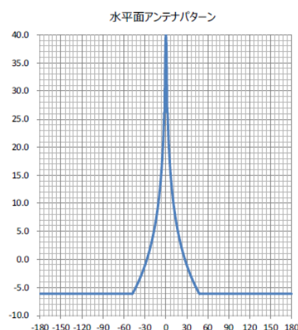
図 2. 3. 5. 3-4 FPU の指向性減衰特性
