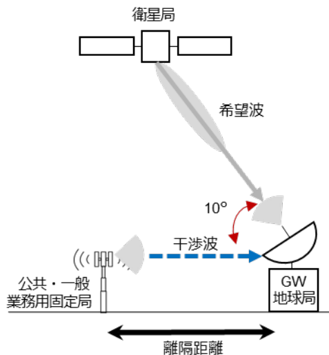
図 2. 3. 3. 5-2 公共・一般業務用固定局から 700MHz 帯非静止衛星通信システム (GW 地球局) への与干渉の実運用モデル
