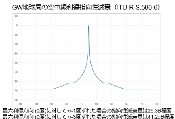
図 2. 1. 3. 2-2 GW 地球局の空中線利得指向性減衰
