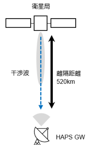
図 2. 3. 9. 3-1 700MHz 帯非静止衛星通信システム（衛星局）から HAPS GW 局への与干渉の対向モデル
