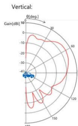
図2. 2. 3. 1-2 ITS 車載器の指向性減衰特性(垂直)
