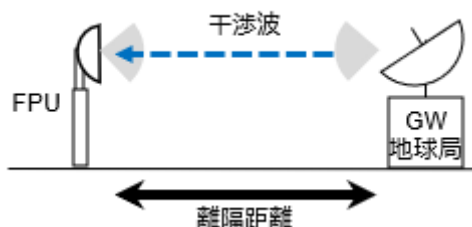
図 2. 3. 5. 3-1 700MHz 帯非静止衛星通信システム (GW 地球局) から FPU への干渉の対向モデル
