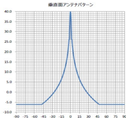
図 2. 3. 5. 2-3 FPU の指向性減衰特性(垂直面)
