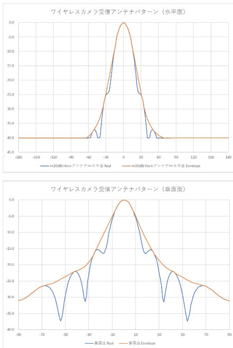
図 2. 3. 6. 1－1 Wireless Camera の指向性減衰特性
