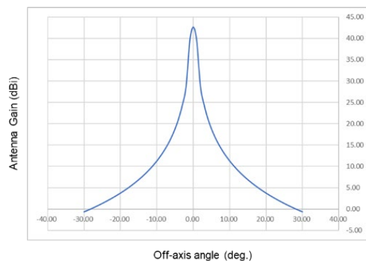
図 2. 3. 3. 2－3 公共・一般業務用固定局の指向性減衰特性(垂直面)
