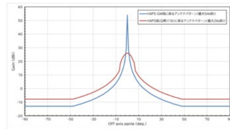
図 2. 3. 9. 4-4 HAPS 局の指向性減衰特性
