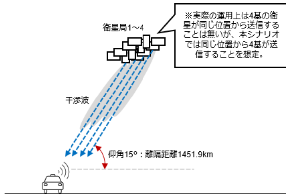
図 2. 2. 3. 2-7 衛星局（仰角 15 度）から ITS 車載器（隣接）への干渉共用検討モデル
