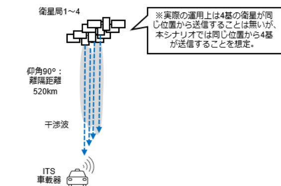
図 2. 2. 3. 2-5 衛星局（仰角 90 度）から ITS 車載器（隣接）への与干渉共用検討モデル
