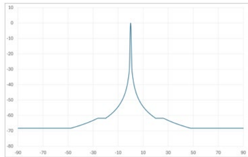
図 2. 3. 10. 13-3 GW 地球局の指向性減衰特性
