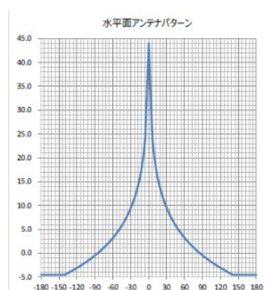
図 2. 3. 4. 3-4 無線アクセス局の指向性減衰特性
