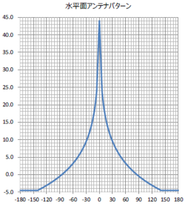
図 2. 3. 4. 5-4 無線アクセス局の指向性減衰特性
