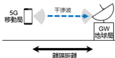
図 2. 3. 2. 5-1 5G 移動局から 700MHz 帯非静止衛星通信システム (GW 地球局) への与干渉の対向モデル
