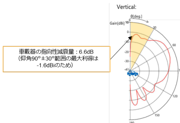
図 2. 2. 3. 2-6 ITS 車載器の指向性減衰特性(垂直面)
