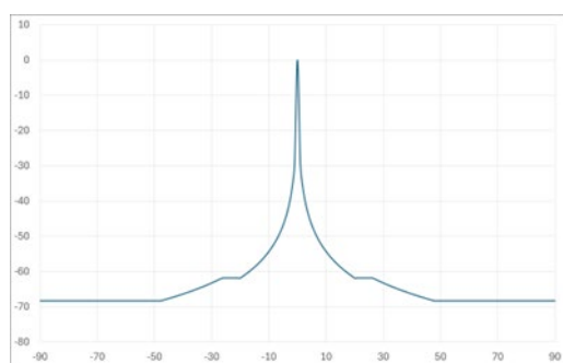
図 2. 3. 4. 3-3 GW 地球局の指向性減衰特性
