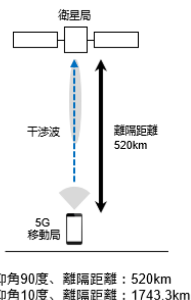
図 2. 3. 2. 4－1 5G 移動局から 700MHz 帯非静止衛星通信システム（衛星局）への与干渉の対向モデル
