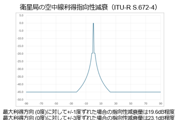
図 2. 1. 3. 2-1 衛星局の空中線利得指向性減衰
