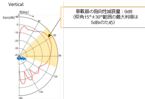
図 2. 2. 3. 2-8 ITS 車載器の指向性減衰特性(垂直面)
