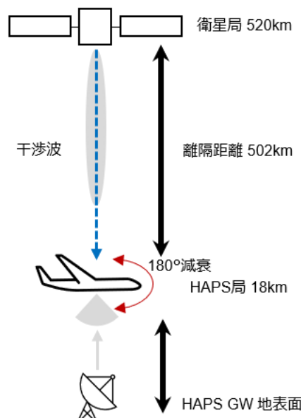
図 2. 3. 9. 2-2 700MHz 帯非静止衛星通信システム（衛星局）から HAPS 局への与干渉の実運用モデル
