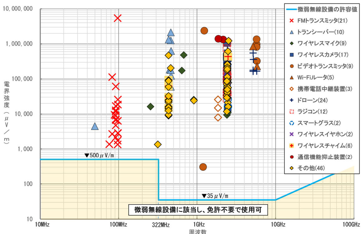
図：令和7年度無線設備試買テスト結果 (用途別の微弱無線設備の基準適合状況)
