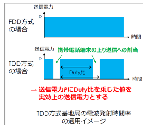
図4 TDD方式基地局の電波発射時間率の適用イメージ( F_{TDC} の参考) 出典：第9回基地局等評価方法作業班 資料9-1
