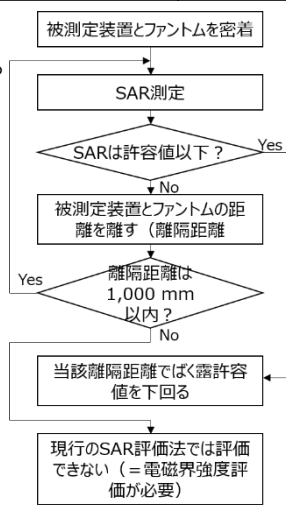
図2 測定フロー
