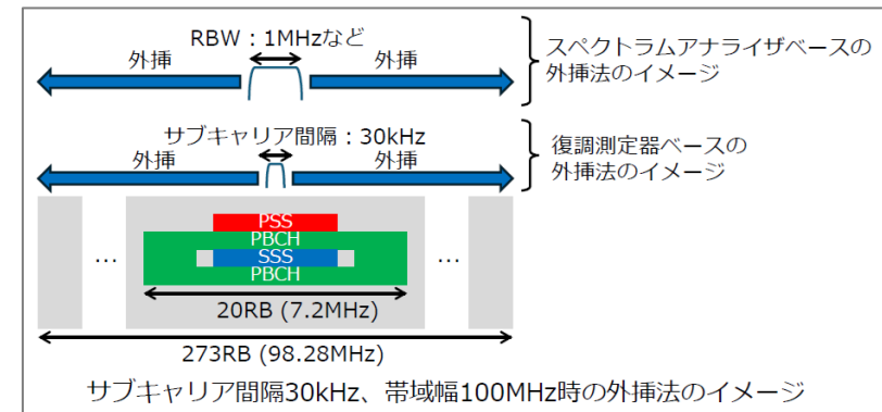
図6 外挿法のイメージ
