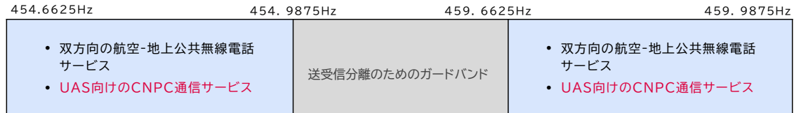
図 31 450-470 MHz 帯におけるチャンネルプラン 42
