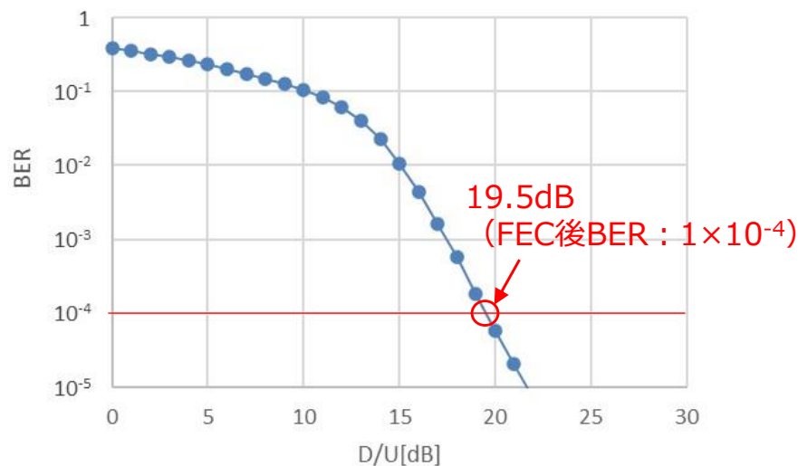
BER特性
