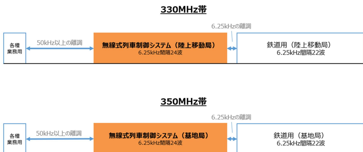
図 1-5 300MHz 帯無線式列車制御システム使用周波数帯
