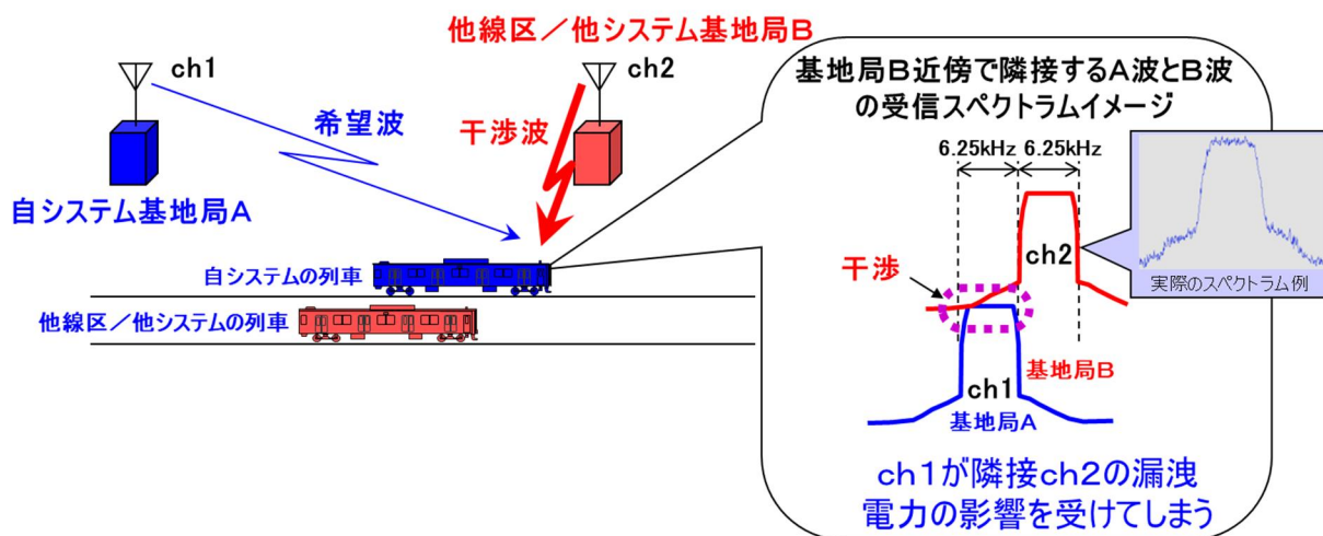
図 2-4 隣接チャンネル干渉のイメージ
