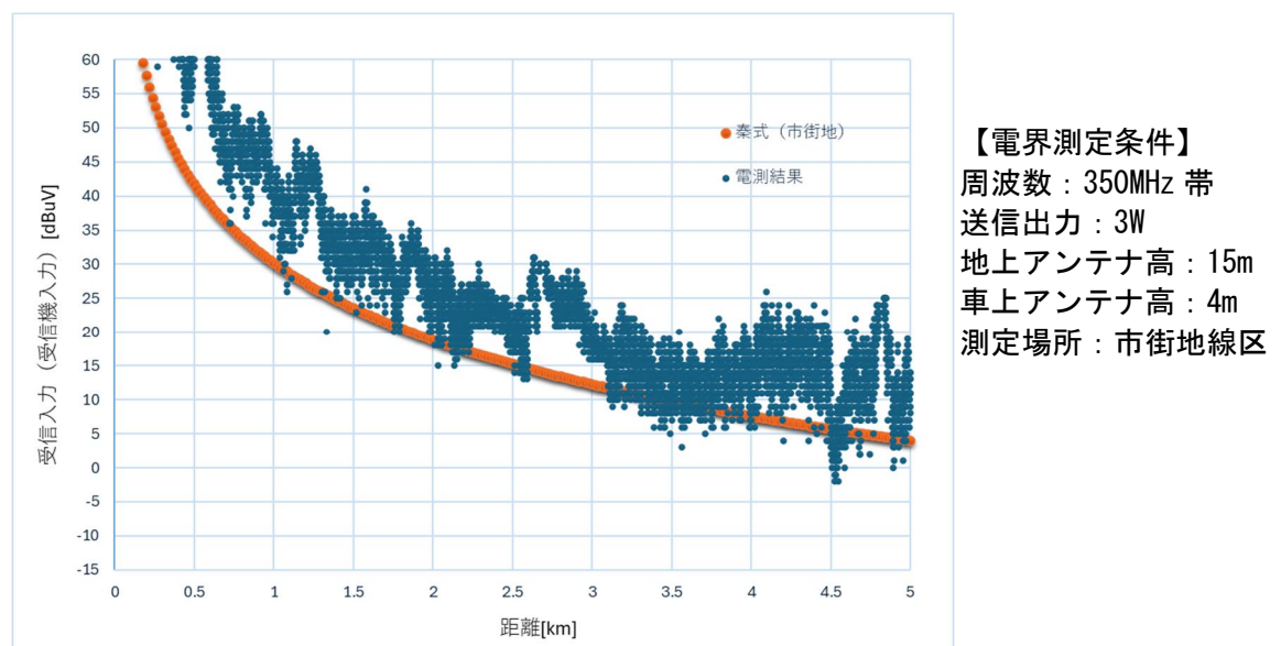
図 1：秦式電波伝搬特性（市街地）と電界測定結果
