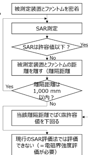
図2 測定フロー
