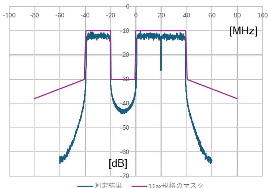
図 3-19 レガシー端末：80 MHz 送信時の 20 MHz パングチャリングの測定結果
