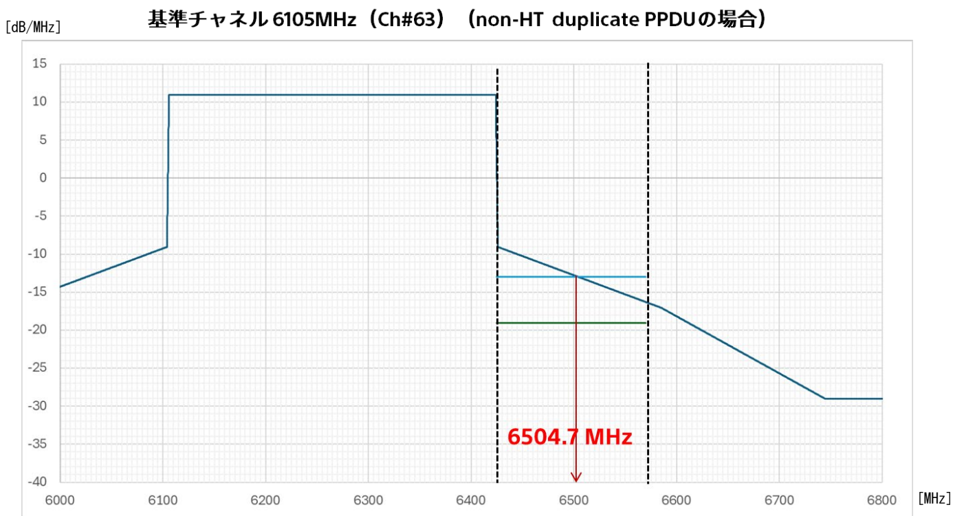
図 2 - 30 : 320 MHz BW の場合 (6425 MHz 超 6570 MHz 未満の領域)
