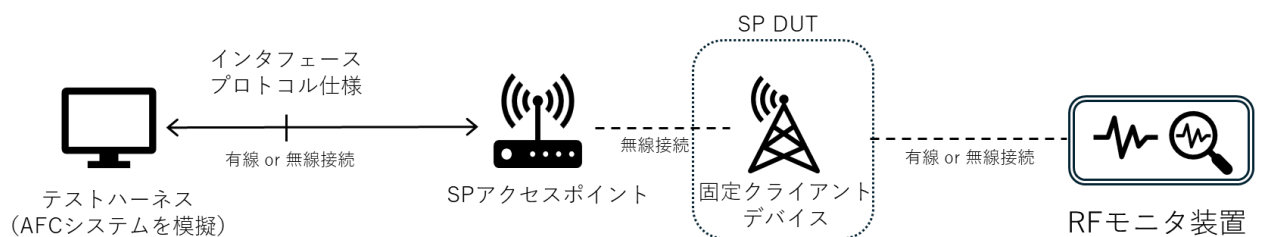
図2-33：SP モードデバイス（固定クライアントデバイス）の適合性検査の構成
