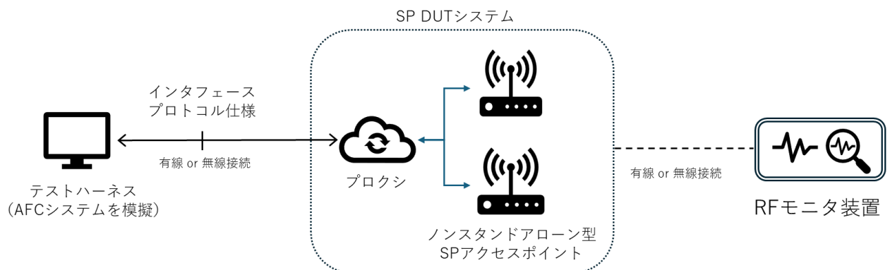
図2-32：SP モードデバイス（ノンスタンドアローン型アクセスポイント）の適合性検査の構成
