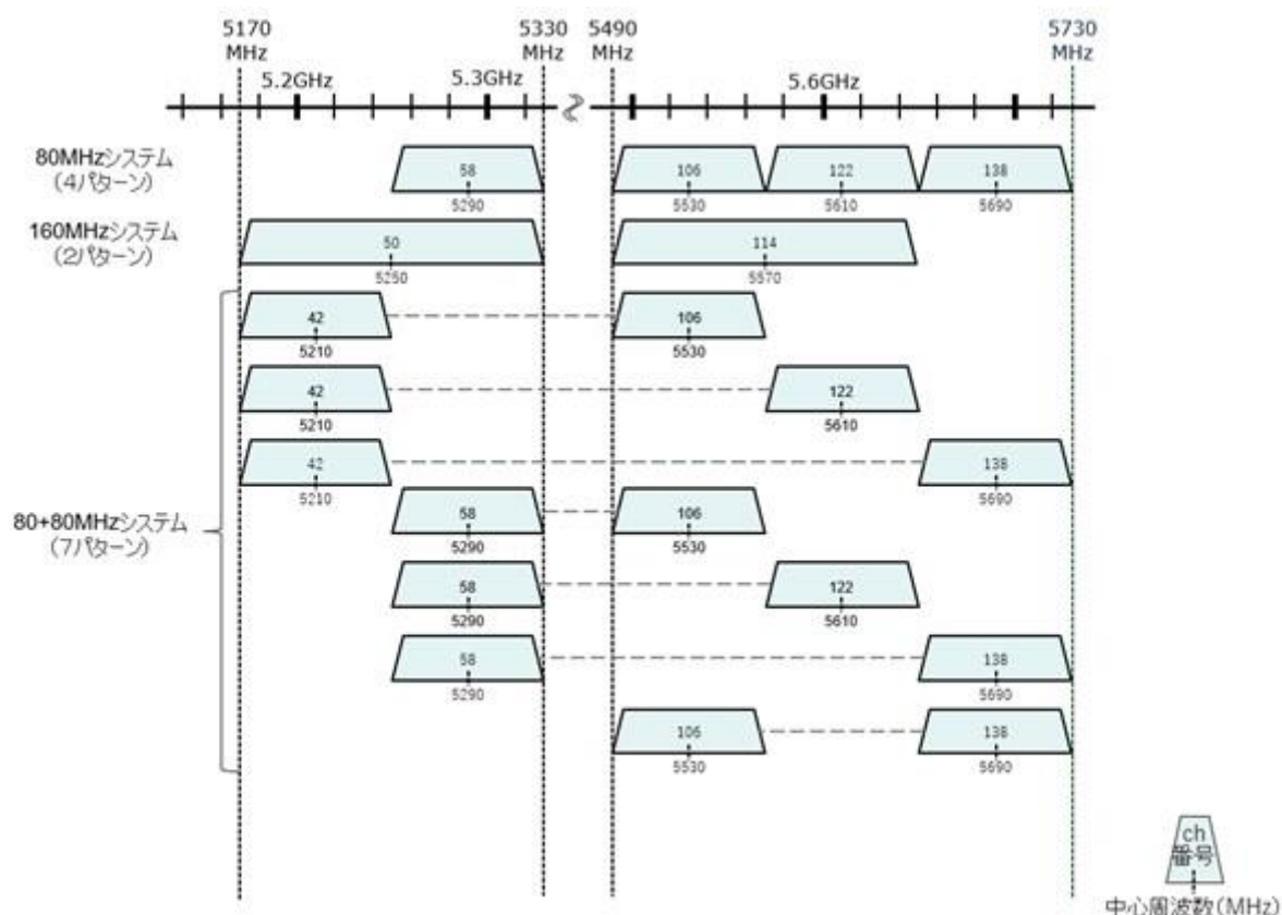
図 3-18 パルクチャリングが適用可能な 5.2/5.3/5.6 GHz 帯のチャネル配置
