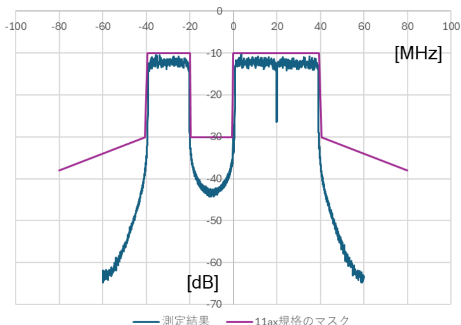
図 3-19 レガシー端末：80 MHz 送信時の 20 MHz パンクチャリングの測定結果
