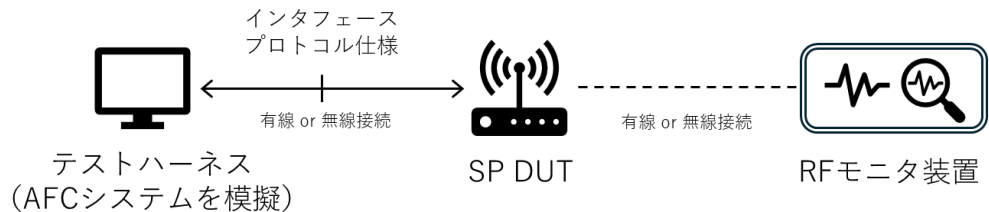
図2-31：SP モードデバイス（スタンドアローン型アクセスポイント）の適合性検査の構成
