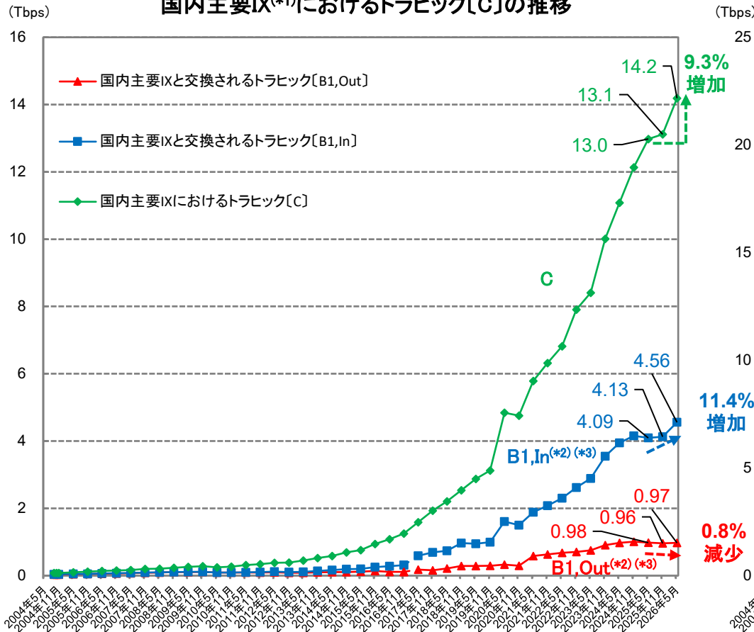
国内主要IX(*1)と交換されるトラフィック[B1] 国内主要IX(*1)におけるトラフィック[C]の推移
