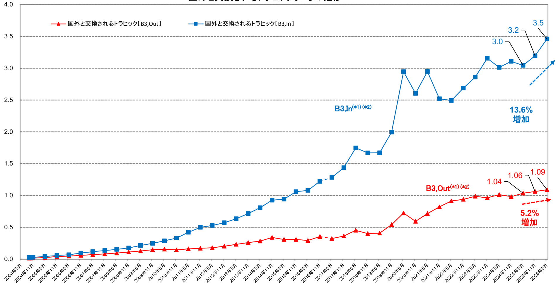
国外と交換されるトラフィック[B3]の推移
