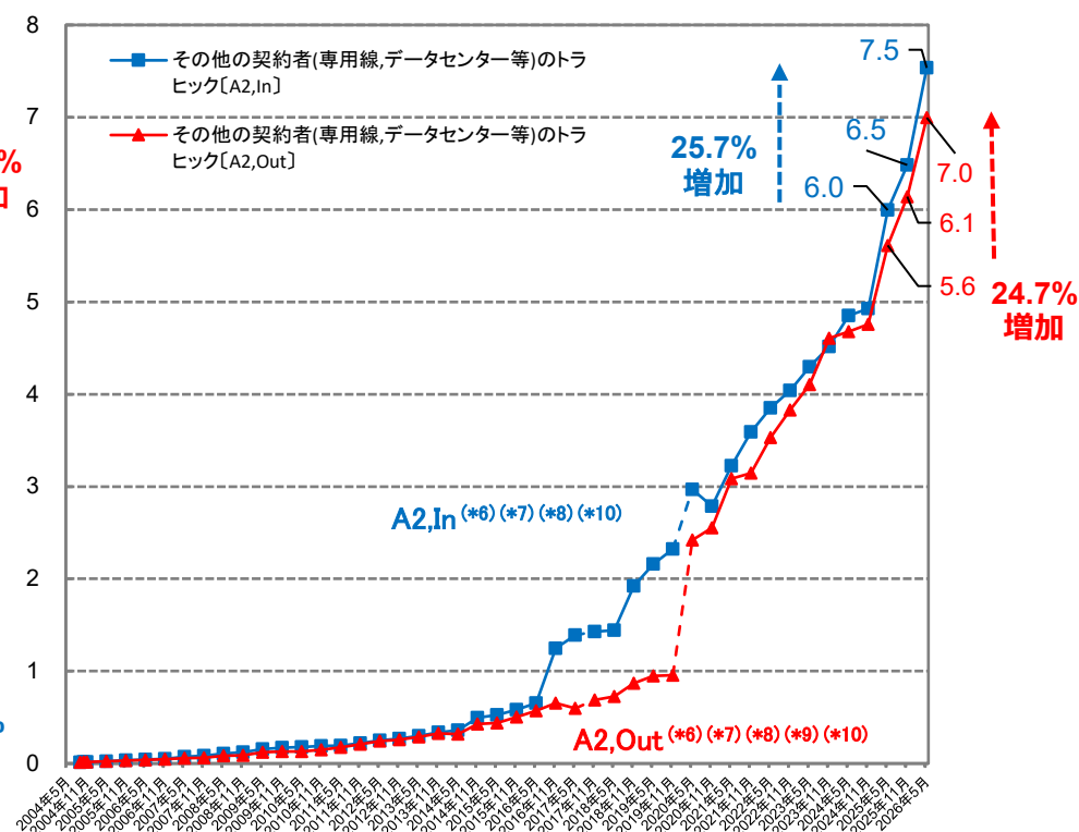
(Tbps) その他専用線等の契約者のトラフィック[A2]の推移
