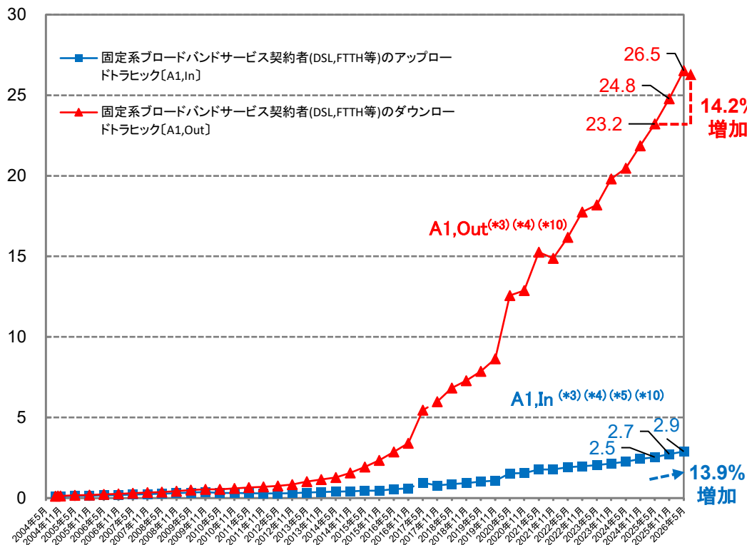
(Tbps) 協力ISPの固定系 broadband サービス契約者のトラフィック[A1]の推移
