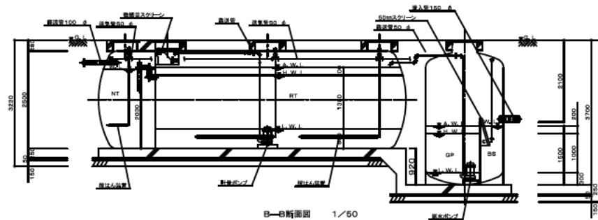
B-B断面図 1/50
