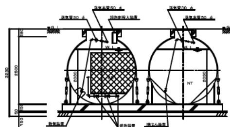
C-C断面図 1/50
