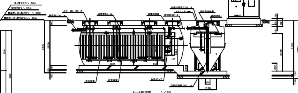
A-A断面図 1/50
