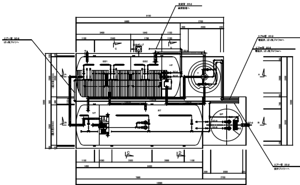
内部平面図 1/50
