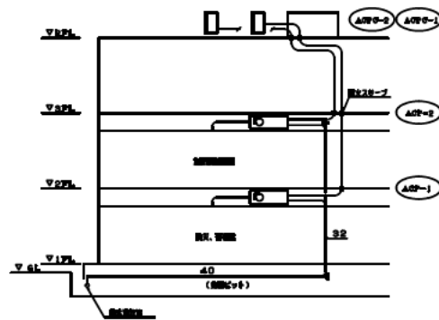
乗務員ルームエアコン配管
