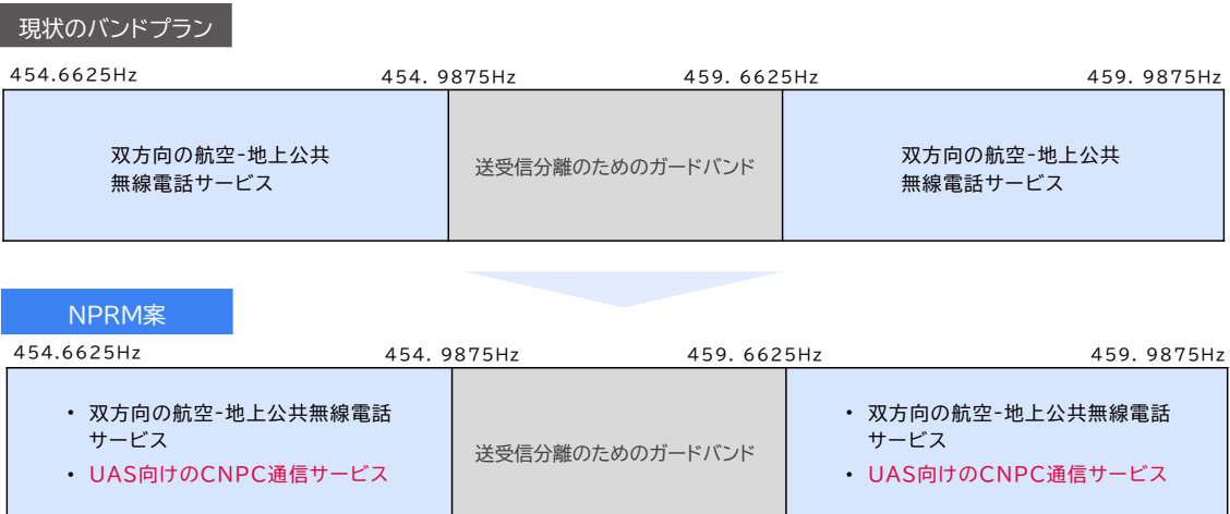
図 31 450-470 MHz 帯におけるチャネルプラン 42
