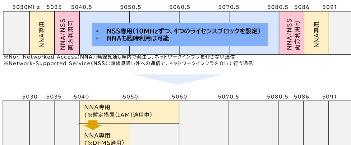
図 29 5030-5091 MHz 帯における UAS 制御用通信チャネル提案 40
