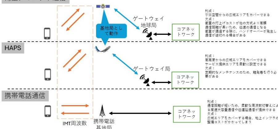
図表 1-16：衛星ダイレクト通信についての詳細
