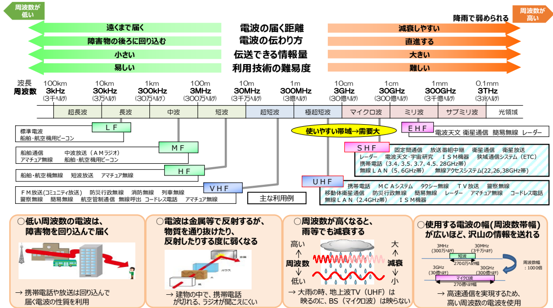
図表 1 電波の特性と利用形態
