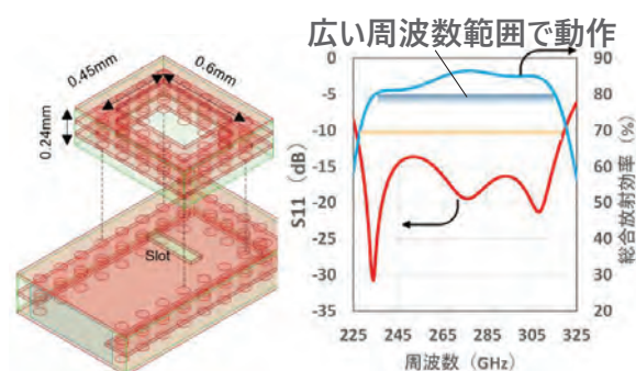
アンテナ設計例
