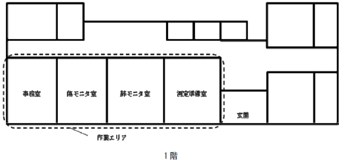
図 2 放射線保健室 平面図
