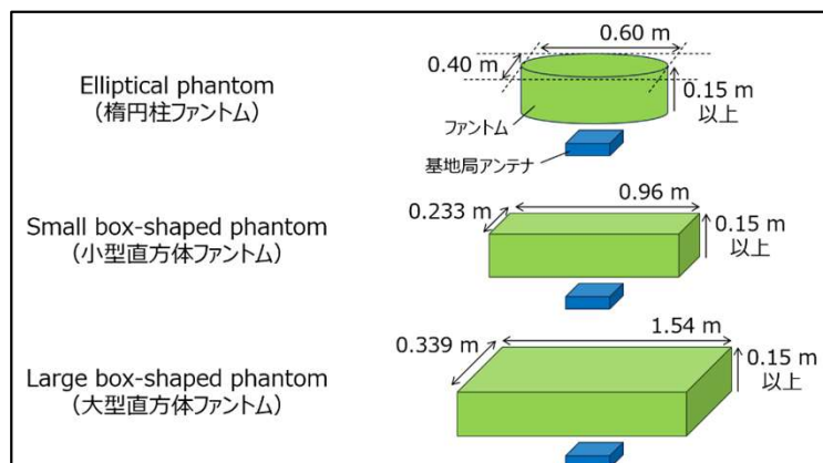
図1 局所SAR・全身平均SARの測定に用いるファントムの形状
