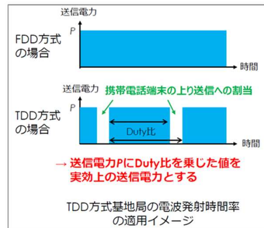
図4 TDD方式基地局の電波発射時間率の適用イメージ ( F_{TDC} の参考)
