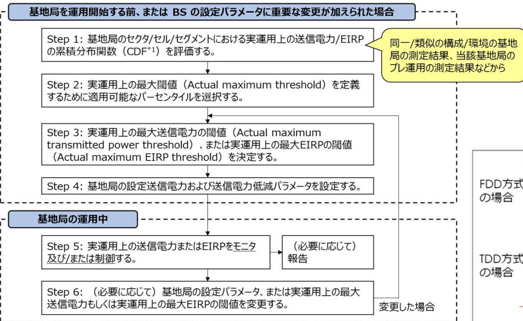
図3 AMP/AMEIRP閾値に基づく製品設置時の適合性確認手順 出典: 第9回作業班 資料9-1
