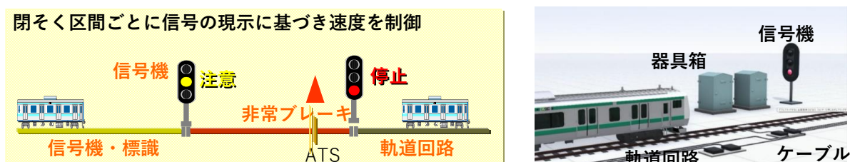
図 1-2 従来の列車制御システム
