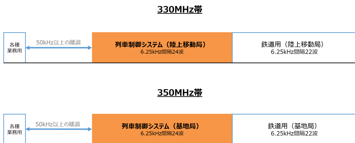
図 1-5 300MHz 帯無線式列車制御システム使用周波数帯
