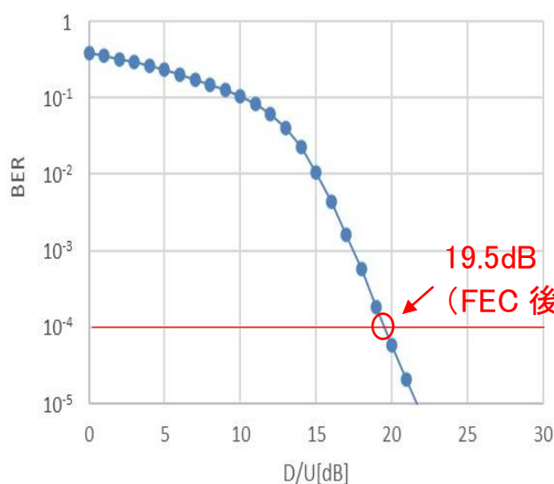
図 2-2 BER-D/U 特性 (新方式×新方式)
