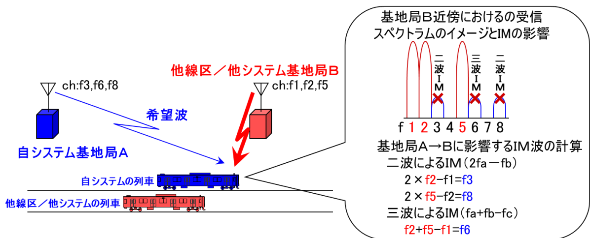
図 2-5 相互変調干渉のイメージ
