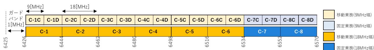
図 4.3.3-2 C バンドのチャンネル配置
