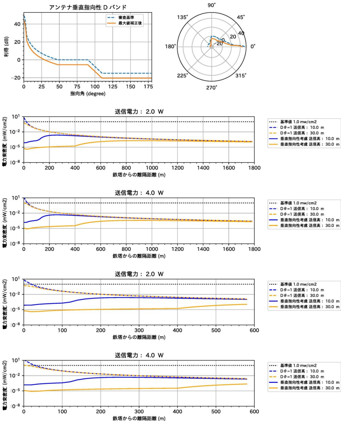
図 2 次世代 TSL 離隔距離と電力束密度の計算例
