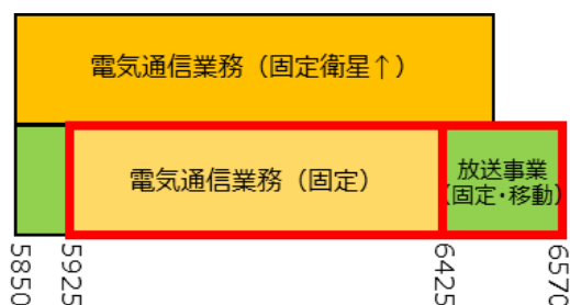
図 4.3.3-1 電気通信業務(固定)の周波数帯
