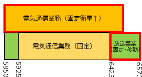
図 4.3.7-1 電気通信業務(固定衛星アップリンク)の周波数帯
