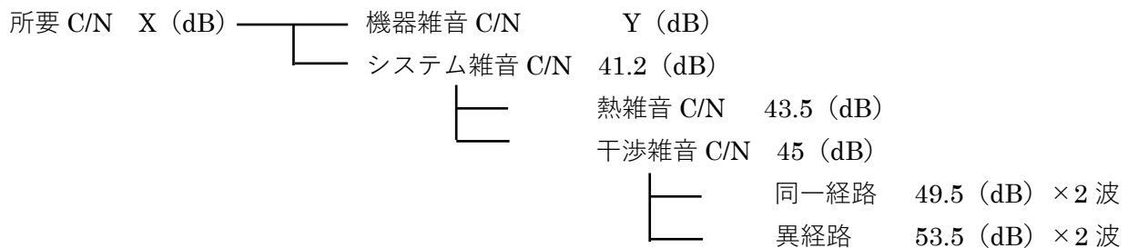
図 5 次世代 IF 伝送方式 C/N 配分(従属同期方式のうち低雑音方式の場合)
