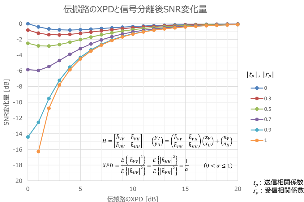
図 1 XPD 低下時の SNR 変化量
