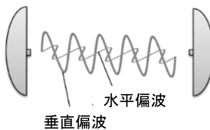
図 2.1.2-4 偏波 MIMO 技術
