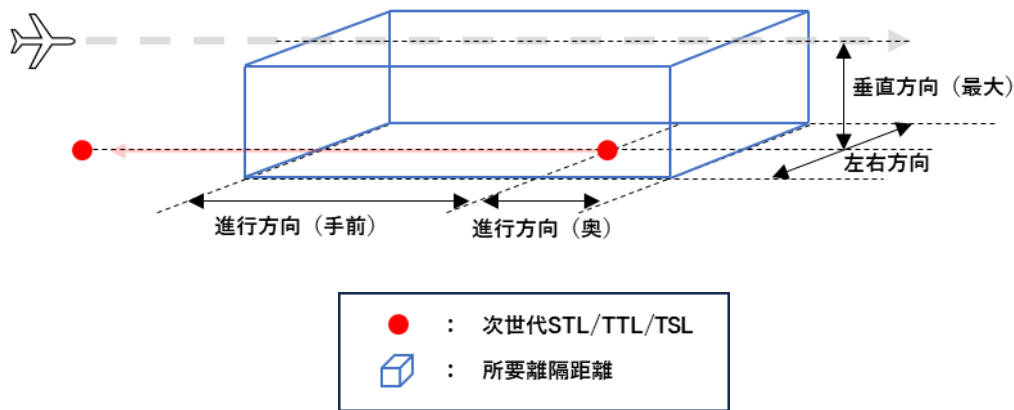
図 4.3.1.2-3 次世代 STL/TTL/TSL と航行用レーダーの所要離隔距離
