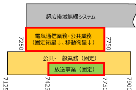
図 4.3.8-1 電通・公共業務(固定衛星ダウンリンク・移動衛星ダウンリンク)の周波数帯
