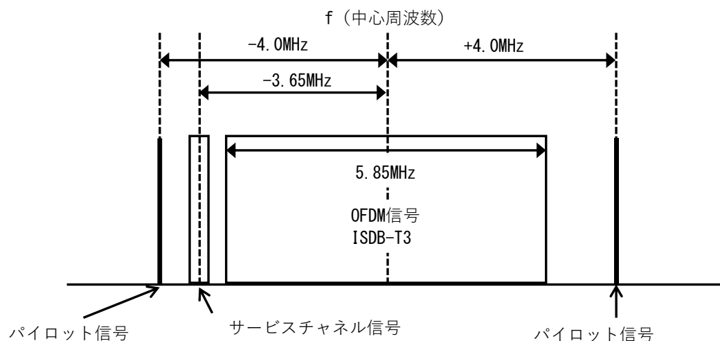
図 2.3.2-1 伝送信号の周波数配置の例
