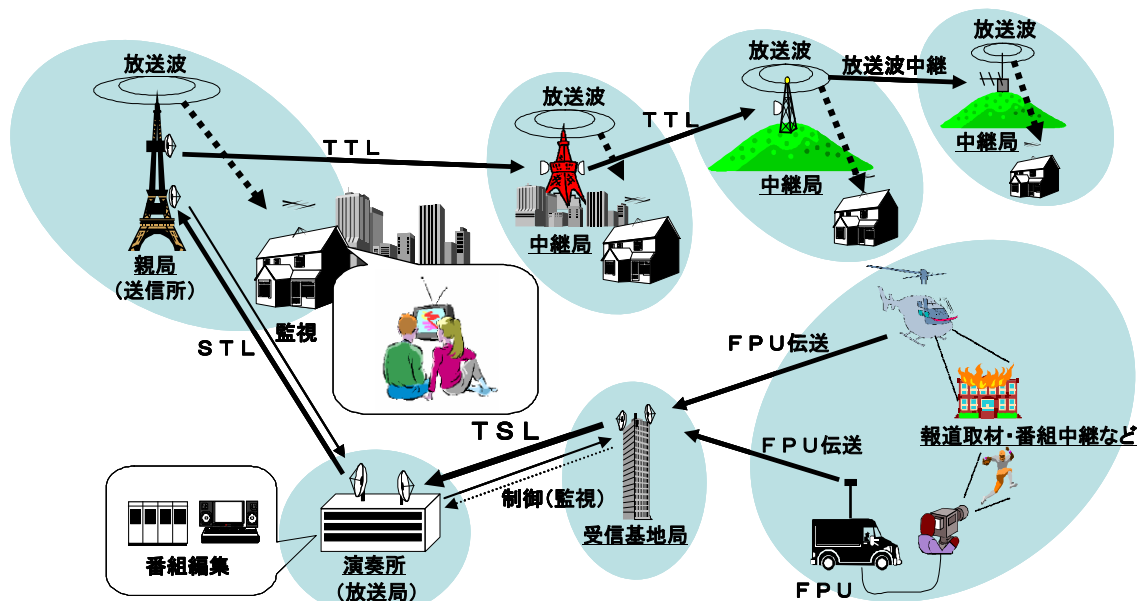
図 1.1-1 テレビジョン放送ネットワーク例
