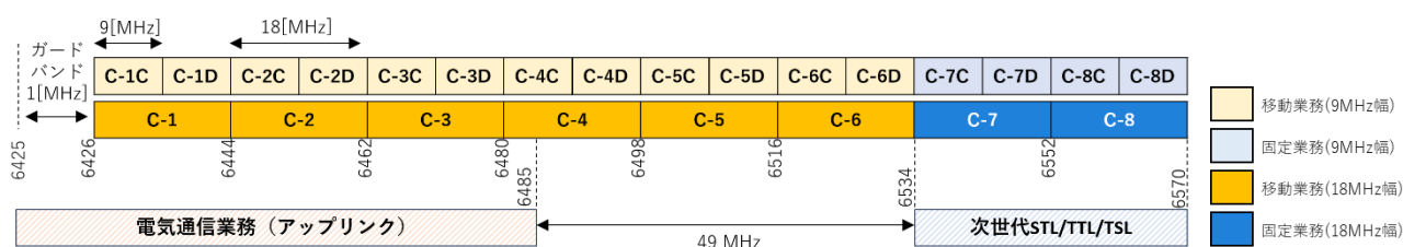
図 4.3.7-2 C バンドのチャネル配置
