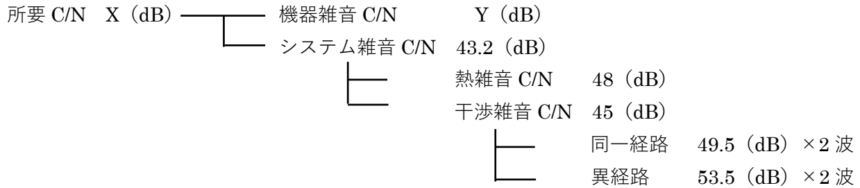
図 4 次世代 IF 伝送方式 C/N 配分(従属同期方式のうち低雑音方式以外の方式)
