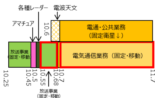
図 4.3.6-1 電気通信業務(固定・移動)の周波数帯
