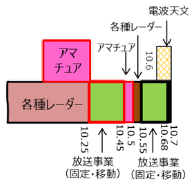
図 4.3.2-1 共用検討におけるアマチュア無線の周波数帯
