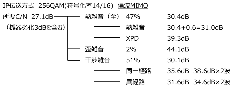
図 3 IP 伝送方式の偏波 MIMO における C/N 配分
