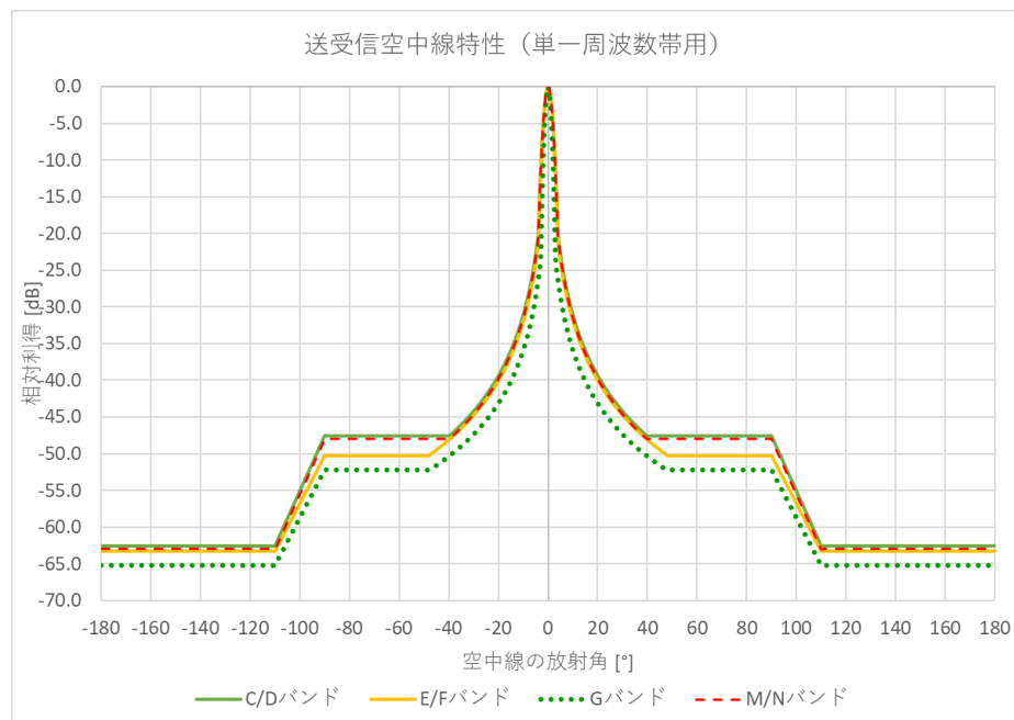
図 4.2.1-1 次世代 STL/TTL の空中線特性
