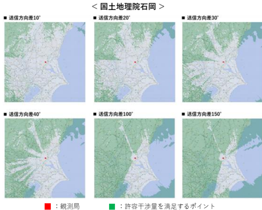
図 4.3.12-8 Fバンドにおける国土地理院石岡の検討結果
