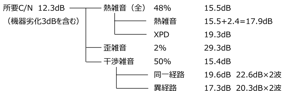
図 5 次世代 TSL 伝送方式(16QAM)の偏波 MIMO における C/N 配分
