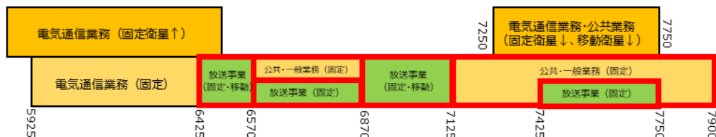
図 4.3.5-1 電通・公共・一般業務(固定)の周波数帯
