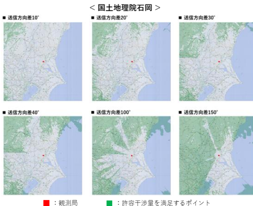
図 4.3.12-7 M バンドにおける国土地理院石岡の検討結果
