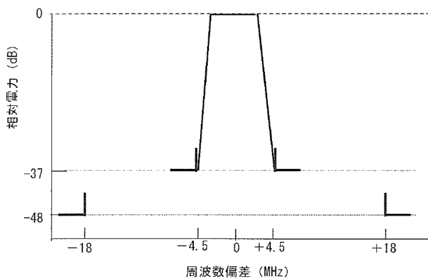
図 1 送信電力スペクトル特性(IP 伝送方式)
