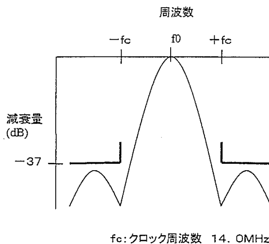
図 1 送信電力スペクトル特性(C/D/E/F/G バンド、ただし C-8 及び D-1 を除く)
