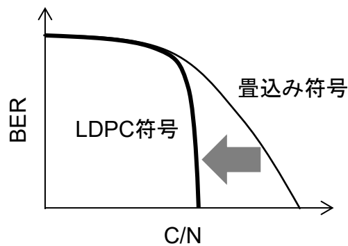
図 3.1.2-3 LDPC 符号の導入
