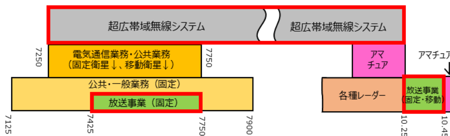
図 4.3.11-1 超広帯域無線システム(UWB)の周波数帯
