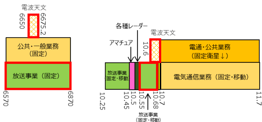
図 4.3.12-1 電波天文(受動)無線システムの周波数帯
