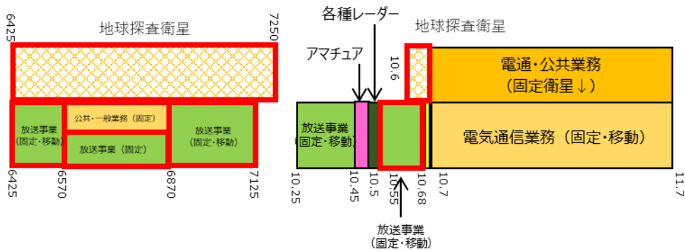
図 4.3.13-1 地球探査衛星業務(受動)の周波数帯
