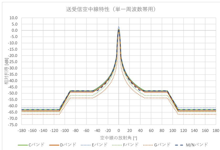
図 4.2.1-2 次世代 TSL の空中線特性
