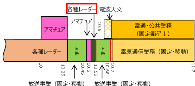
図 4.3.1.1-1 共用検討における各種レーダー(10GHz 帯)との周波数関係
