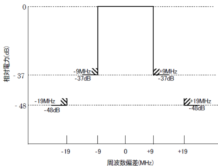
図 2 送信電力スペクトル特性(C-8 及び D-1、M/N バンド)
