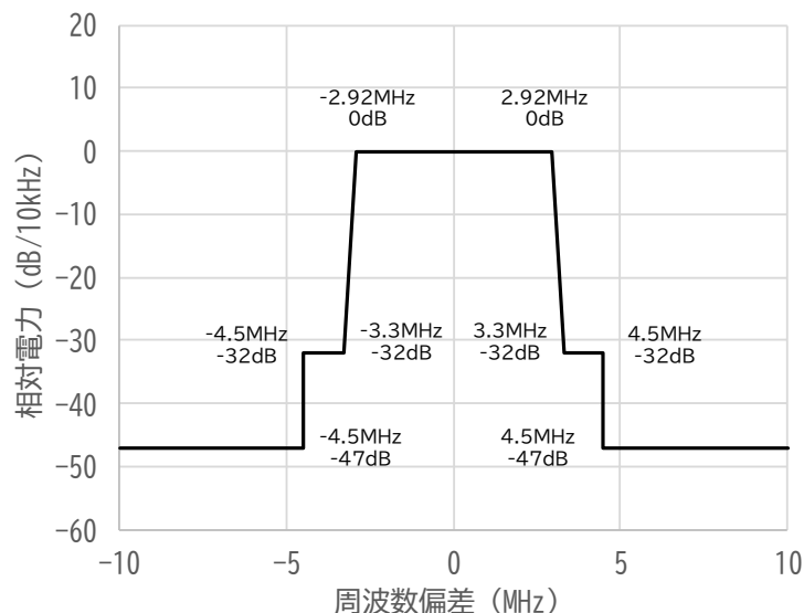
図 1 送信電力スペクトル特性(サービスチャネル信号を使用しない独立同期方式の場合)
