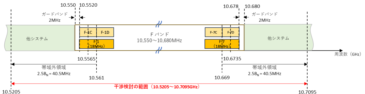
図 4.2.2-1 帯域外干渉の検討範囲(F バンドの例)
