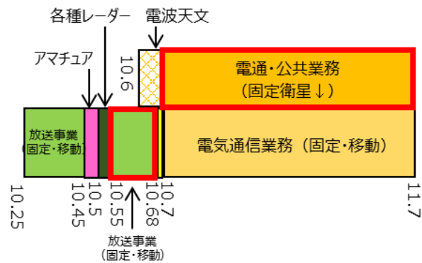
図 4.3.9-1 電通・公共業務(固定衛星ダウンリンク)の周波数帯
