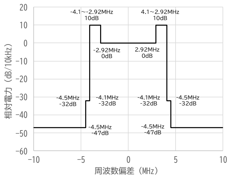
図 2 送信電力スペクトル特性(サービスチャネル信号を使用する独立同期方式の場合及び従属同期方式(低雑音方式を除く)の場合)
