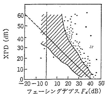
図2 フェージング深さとXPDの相関例
