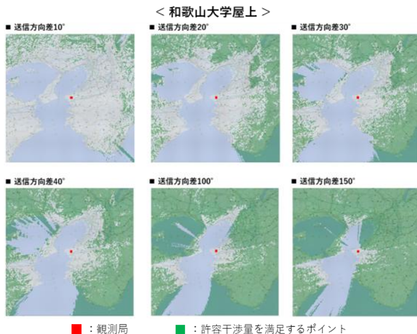
図 4.3.12-6 M バンドにおける和歌山大学屋上の検討結果
