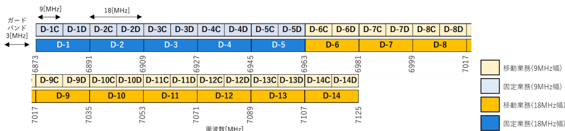
図 4.3.5-2 D バンドのチャンネル配置
