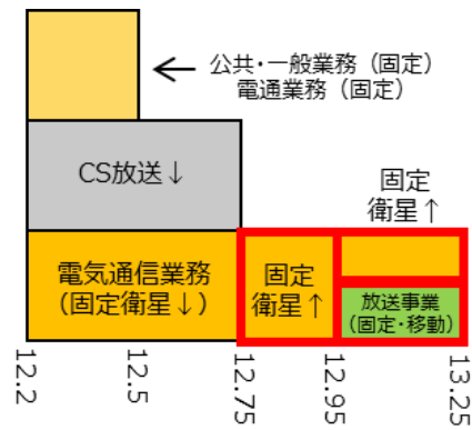
図 4.3.10-1 電気通信業務等(固定衛星アップリンク)の周波数帯
