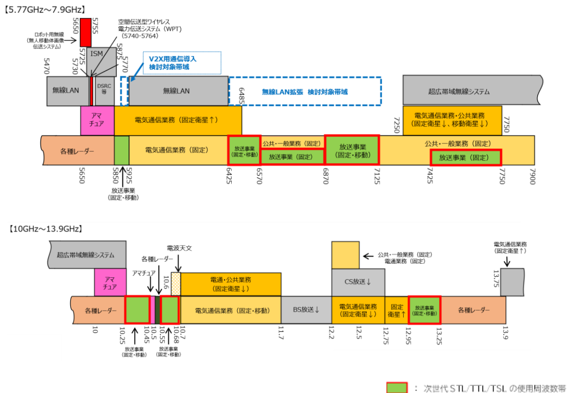
図 4.1-1 次世代 STL/TTL/TSL の使用周波数と他の無線システムの割当て状況
