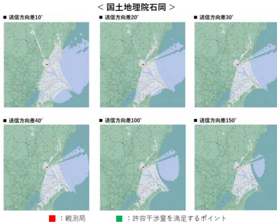
図 4.3.12-9 Fバンドの隣接帯域における国土地理院石岡の検討結果
