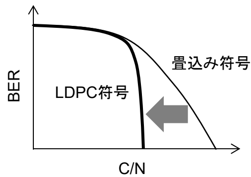
図 2.1.2-2 LDPC 符号
