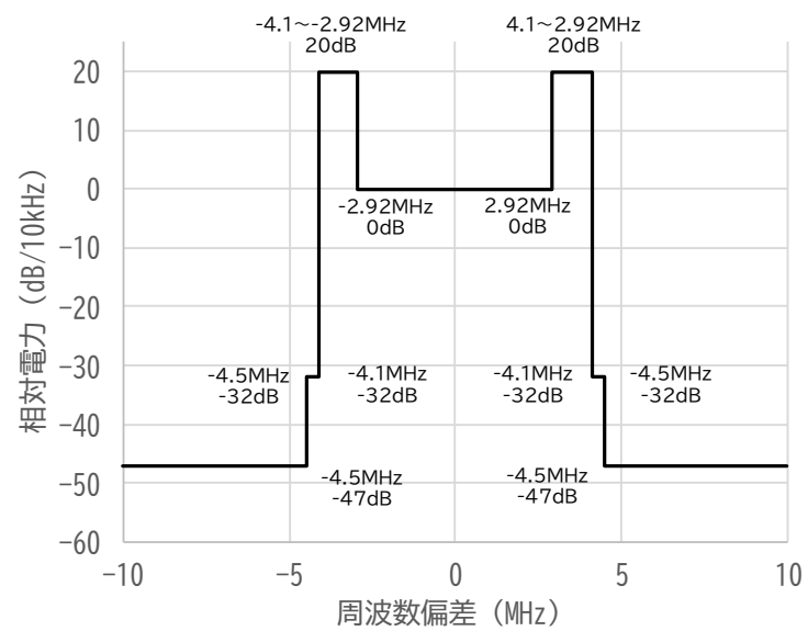
図 3 送信電力スペクトル特性(従属同期方式(低雑音方式)の場合)
