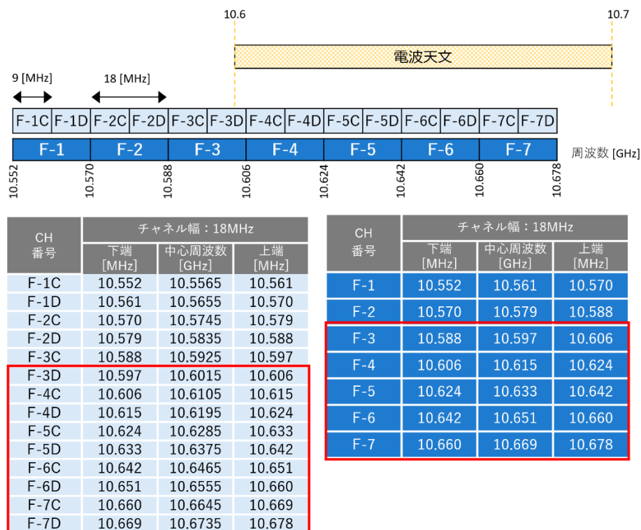
図 4.3.12-3 F バンドにおける放送事業用チャンネルと電波天文の周波数関係
