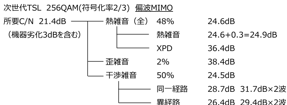
図 4 次世代 TSL 伝送方式(16QAM 以外)の偏波 MIMO における C/N 配分
