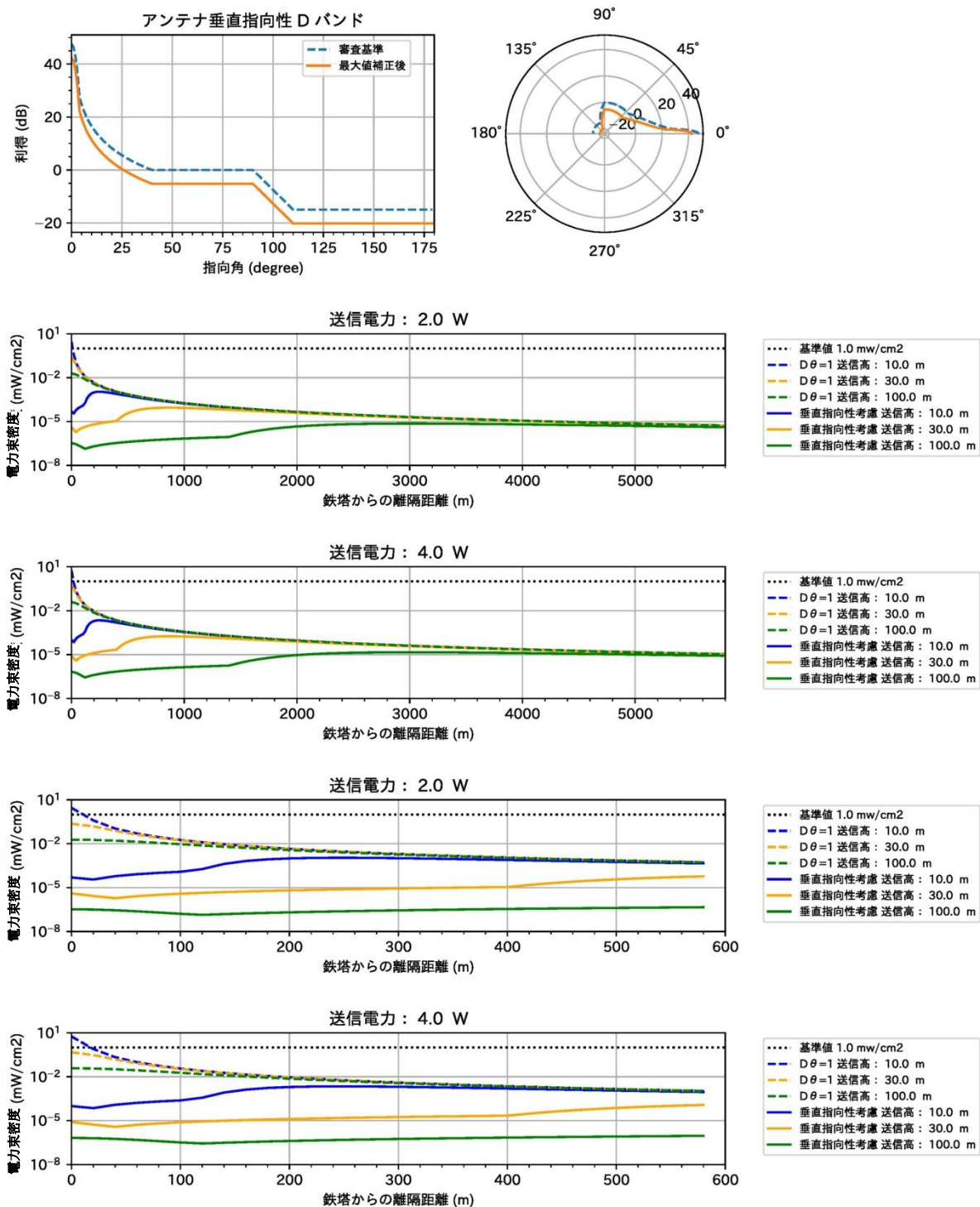
図 1 次世代 STL/TTL 離隔距離と電力束密度の計算例
