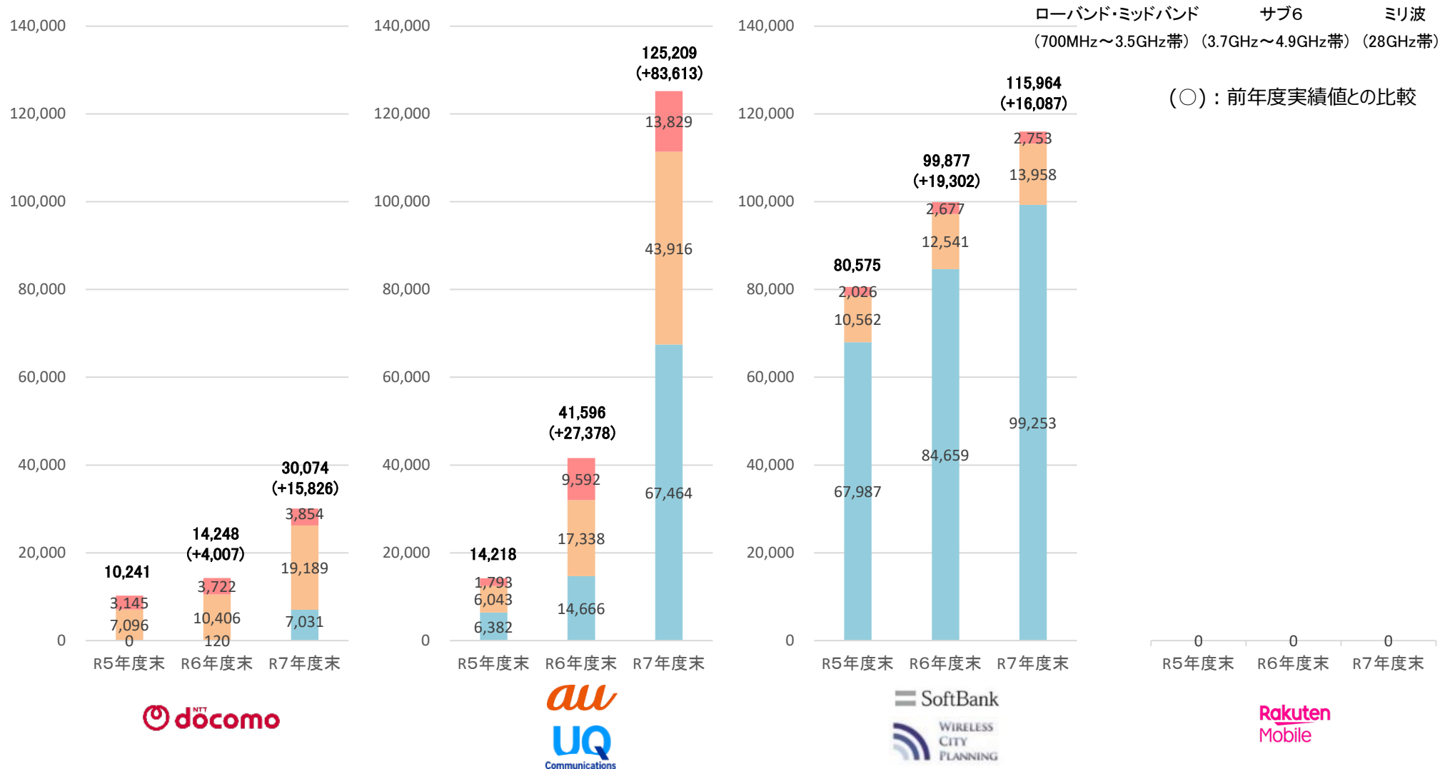
携帯電話事業者（全国BWA事業者を含む。）ごとのSA方式の5G基地局数の推移
