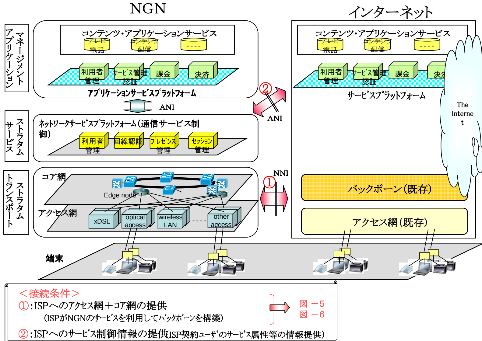
〔図－４〕NTTフィールドトライアルで明示されたサービス・システム・事業構造(レイヤ構造)と 現行インターネットとの関係を示す図
