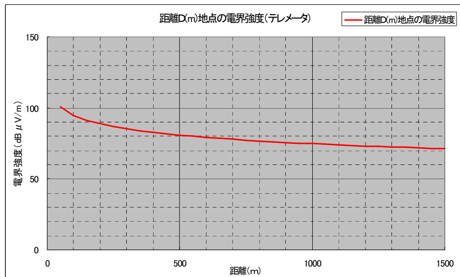
図6-1: 広帯域テレメーターの送受信距離に対する電界強度の計算値(自由空間基本伝搬損失)
