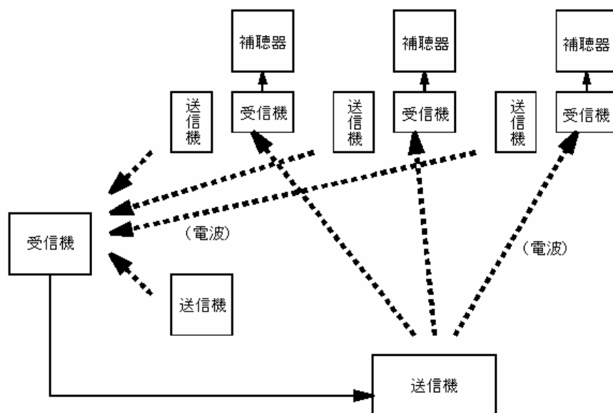
図 2-8: 利用形態⑧ー相互通話方式 3 (双方向電波式)
