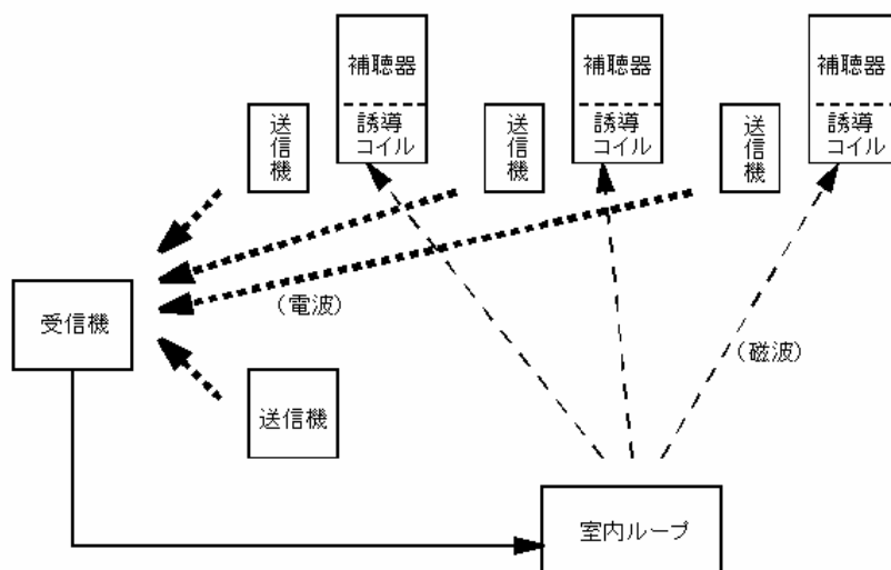
図 2-6: 利用形態⑥ー相互通話方式 1（室内ループ併用式）
