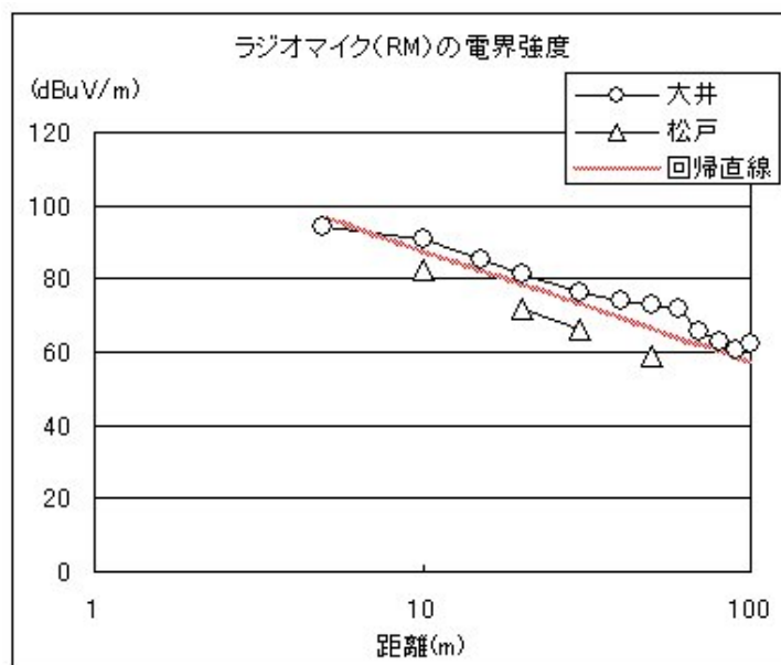
図 7-1: 169MHz 帯補聴援助用ラジオマイク(供試サンプル機)の送受信距離に対する電界強度。—△—は TELEC 松戸試験所における第 1 回実験の垂直偏波のデータ。—○—は大井埠頭中央海浜公園での第 4 回実験(垂直偏波)。——— は△と○に対する回帰直線。
