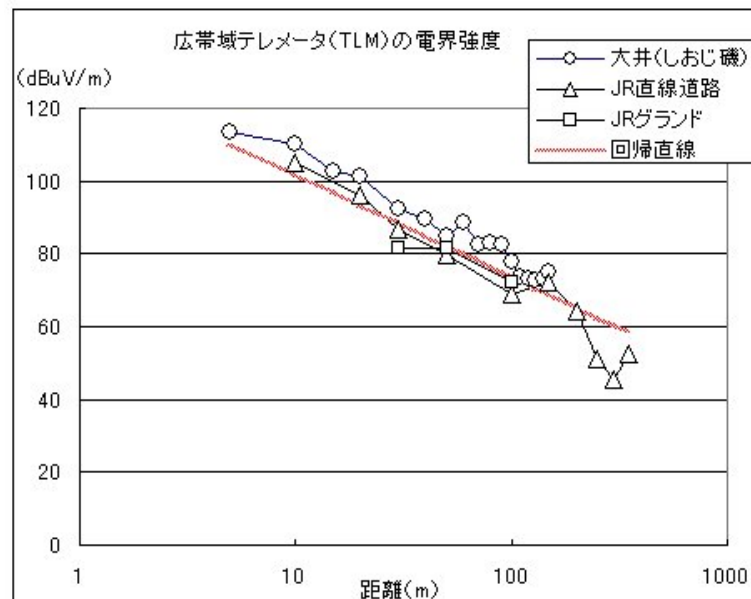
図 7-3: 広帯域テレメーターの距離に対する電界強度。—△— 及び —□— は JR 総研における第 2 回実験のデータ。—○— は大井埠頭中央海浜公園での第 4 回実験。いずれも垂直偏波。— — は全データに対する回帰直線。
