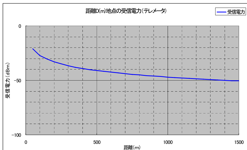
図6-2: 広帯域テレメーターの送受信距離に対する受信電力の計算値(自由空間基本伝搬損失)
