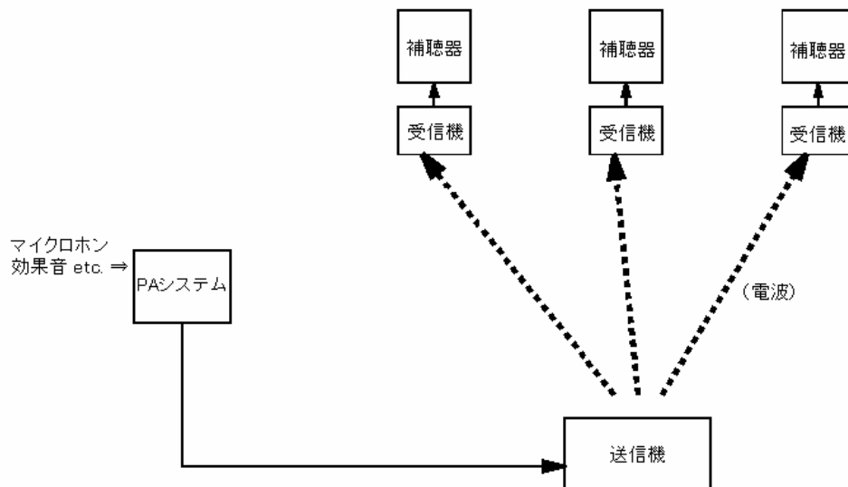
図 2-5: 利用形態⑤ー音響システムの一部となる場合
