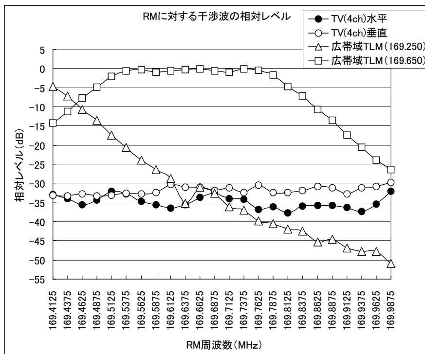
図 7-6: 補聴援助用ラジオマイクの導入を想定している各周波数チャンネル内の干渉波の相対レベル
