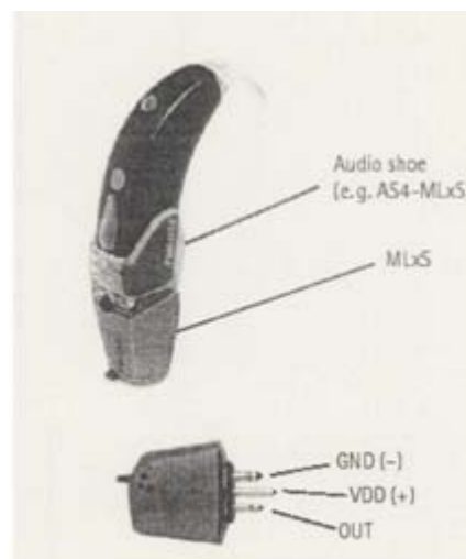
図 5: 耳かけ形補聴器にアタッチするモジュール形式の受信機の一例
