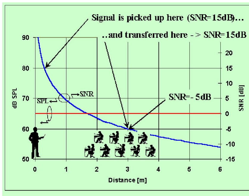
図1 補聴援助システムの効果
