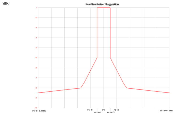
図 2 S 社が提案する将来の変調方式を見込んだスペクトラルマスク
