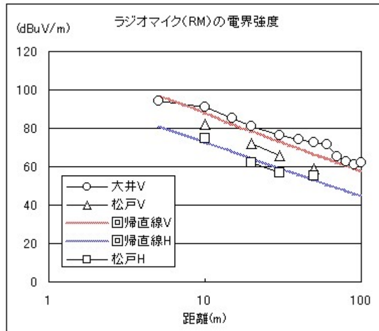
図 4-1: 補聴援助用ラジオマイクの電界強度の距離特性
