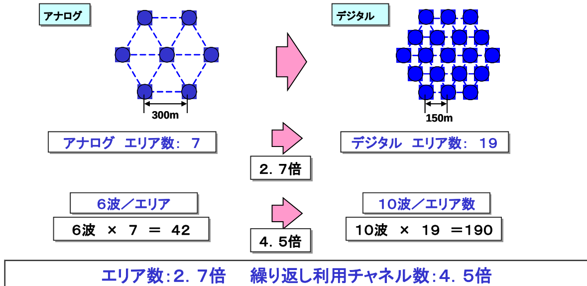
図4 アナログ方式・デジタル方式の同一周波数エリア再利用配置例
