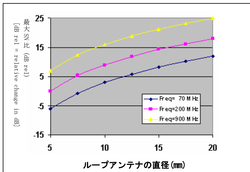
図 2 周波数と小型アンテナの感度の関係
