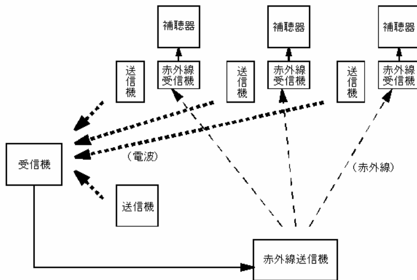
図 2-7: 利用形態⑦ー相互通話方式 2 (赤外線併用式)
