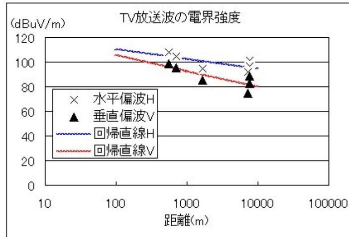
図 7-2: テレビ放送波の放送タワーからの距離に対する電界強度。水平偏波成分 —×— と垂直偏波成分 —▲— を同時に示す。— — と — — はそれぞれの回帰直線。補聴援助用ラジオマイクは垂直偏波を意図している。
