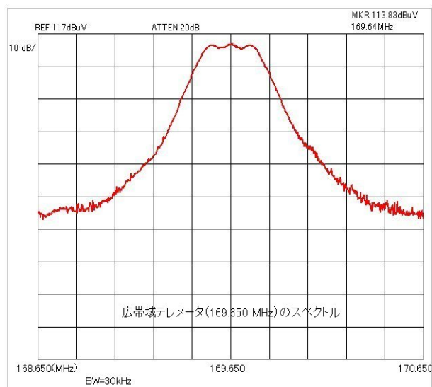
図 7-5: 広帯域テレメーターの周波数スペクトル。
