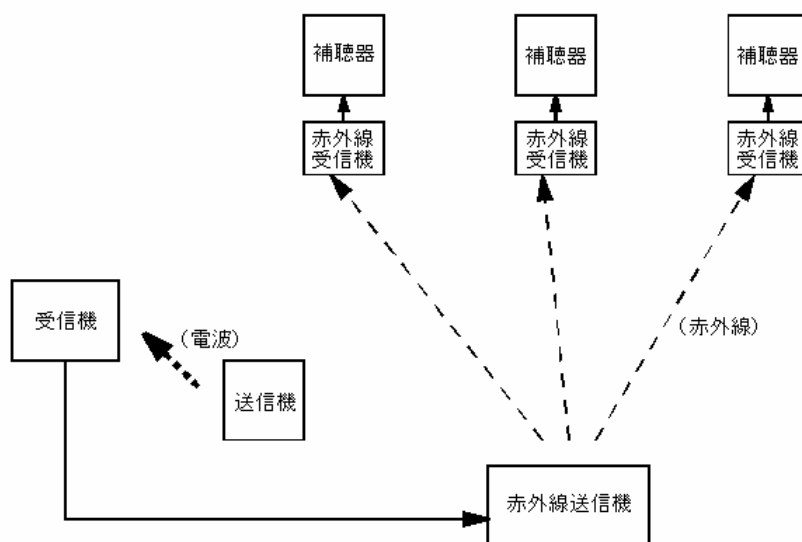
図 2-4： 利用形態④－赤外線併用式
