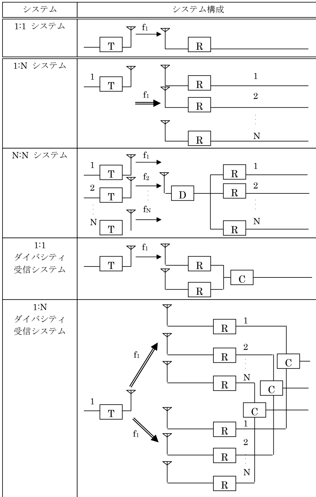
図 デジタル方式B型ラジオマイクのシステム構成例
