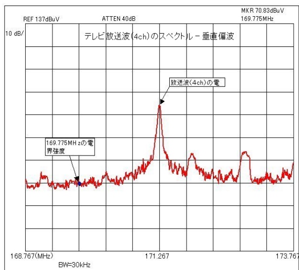
図 7-4: テレビ放送波(4 チャンネル)の周波数スペクトル。分析バンド幅は補聴援助用ラジオマイクの占有周波数帯域幅に近い 30 kHz。
