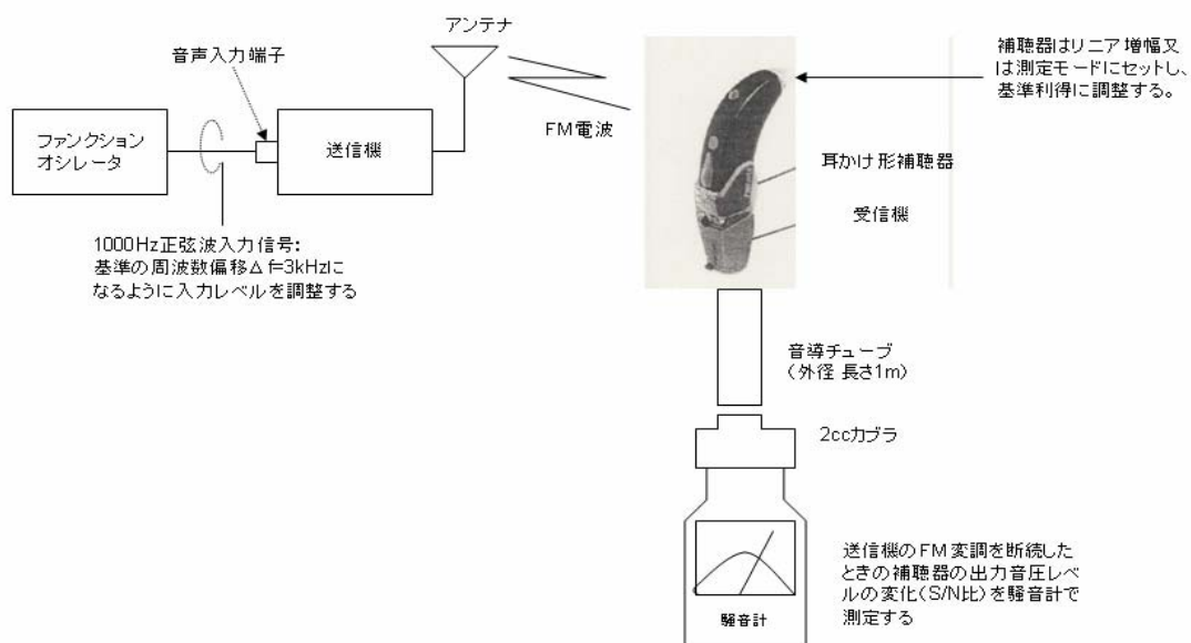
図 7-7： 受信音の信号対雑音比（SN 比）の測定方法。 供試サンプル機（ラジオマイク）の受信機は補聴器に連結する形状である。 送信機より基準の周波数偏移（3kHz）に相当する変調を断続したときの、補聴器の出力音圧レベルの変化を騒音計で測定し SN 比とした。
