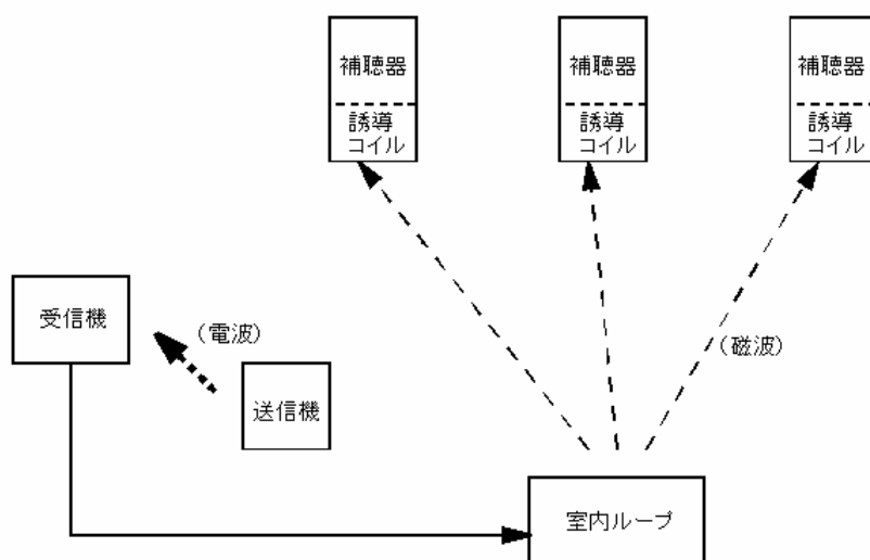
図 2-3： 利用形態③－室内ループ併用式
