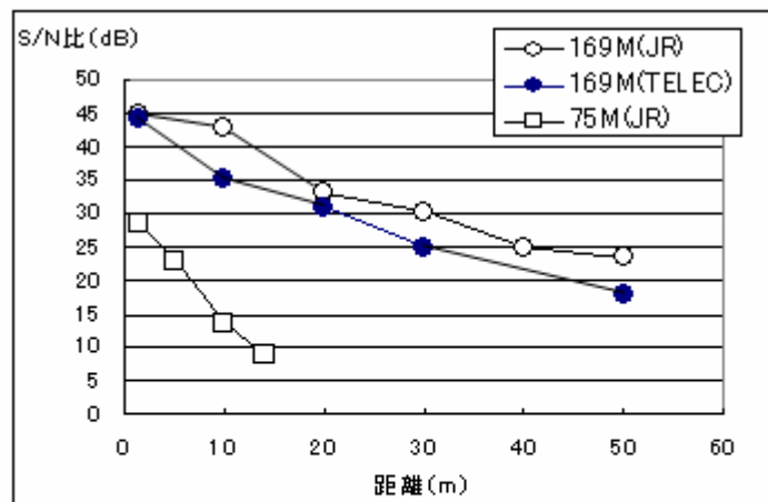
図 6: 補聴援助用ラジオマイク送受信機の通信距離に対する SN 比。JR は 2004 年 8 月 19 日に鉄道総合技術研究所で実施した第 2 回実験の結果を示し、TELEC は 2004 年 6 月 4 日に TELEC 松戸試験所で実施した第 1 回実験の結果を示す。
