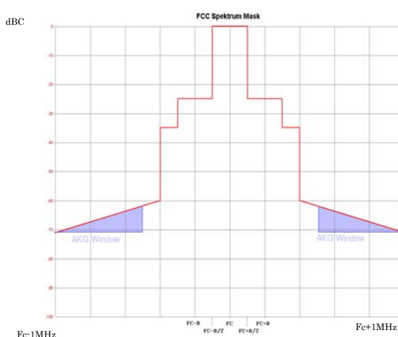
図 1 A 社が提案する次期世界規格としての FCC 規格に近似のスペクトラルマスク
