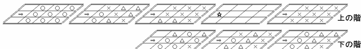
図 8-1: ろう学校教室における同一チャンネルの干渉の状況調査結果 ☆の位置から妨害波を送信したときの、近接する各教室内の9点での干渉の度合いを示す。×＝受信者が干渉波に起因する異音又は雑音を明らかに感知できる、△＝明らかでないが感知できる、○＝感知できない。⇒は各教室の希望波の送信位置（教師の位置）。
