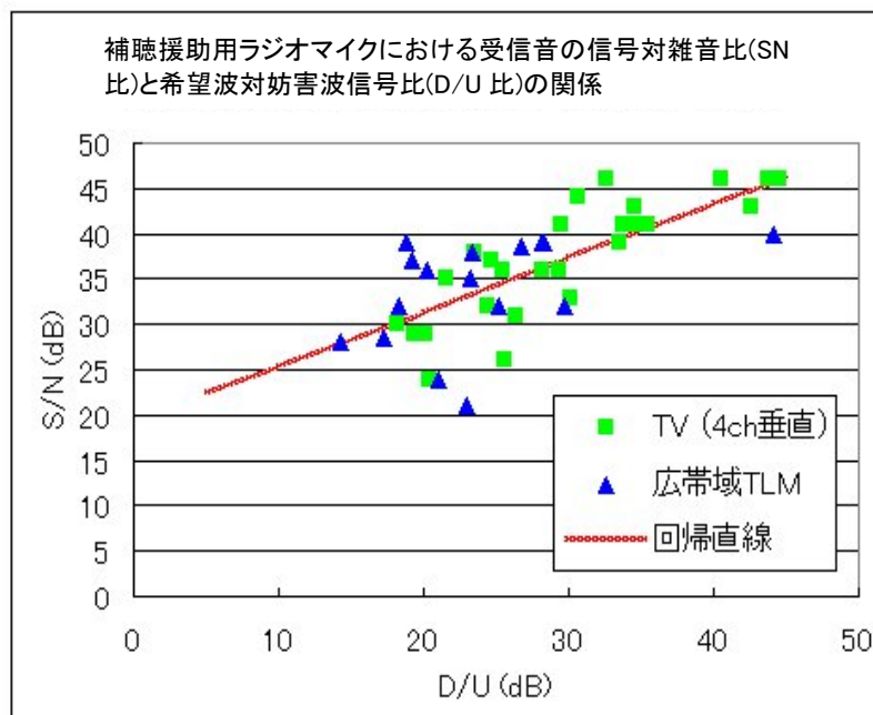
図 7-8: 測定結果に基づく受信音の信号対雑音比(SN 比)と、それに対する希望波対妨害波信号比(DU 比)の関係
