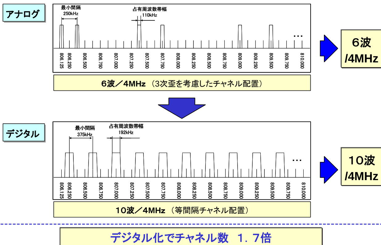
図 2 アナログ方式・デジタル方式の同時使用可能チャネル数の比較
