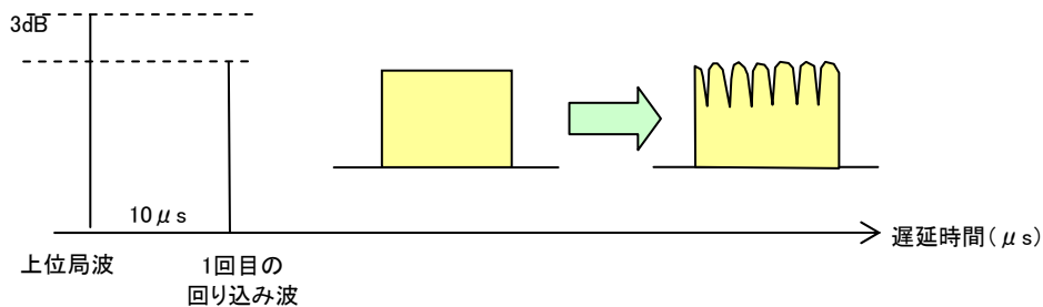
図4. 10 回り込み波が存在する場合の遅延プロフィール（1回、回り込み）
