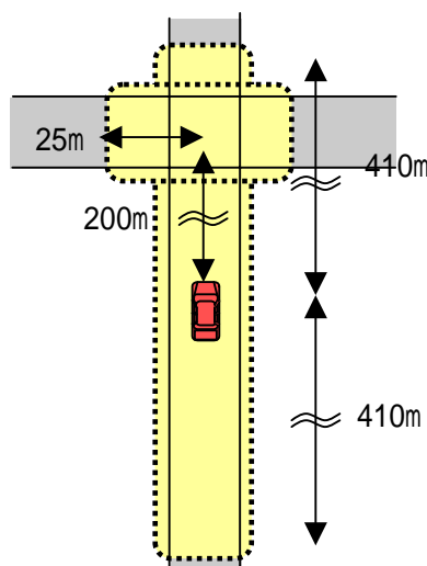
図 17 通信エリア
