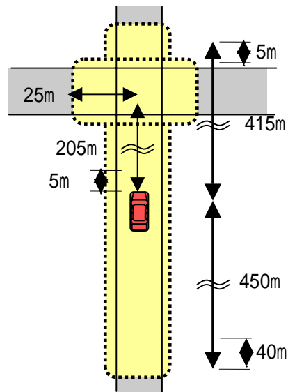
図 30 通信エリア
