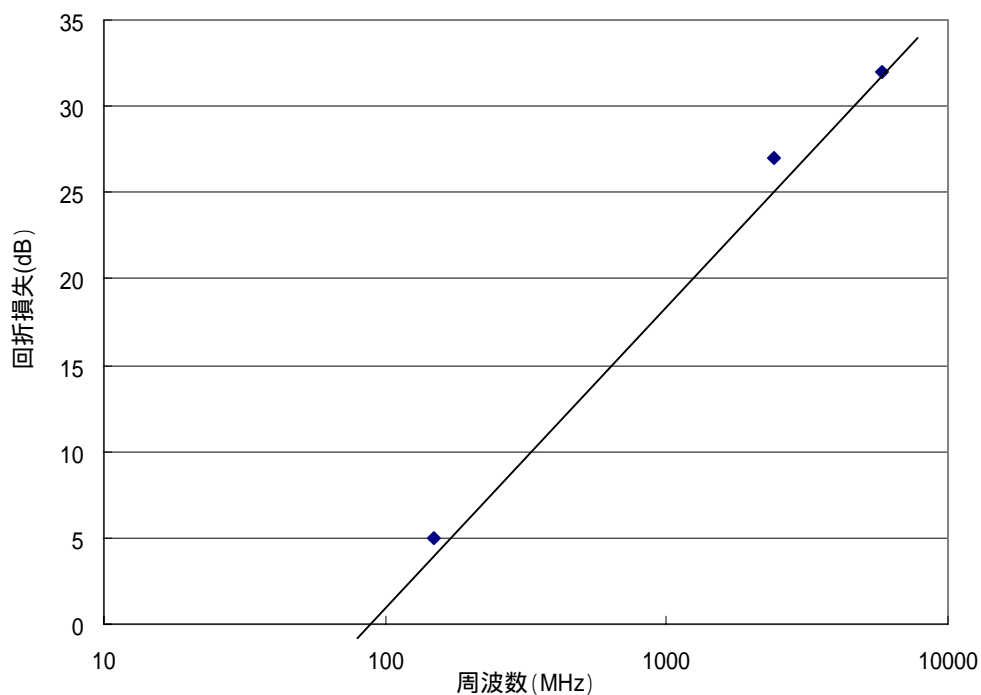
図 22 回折損失
