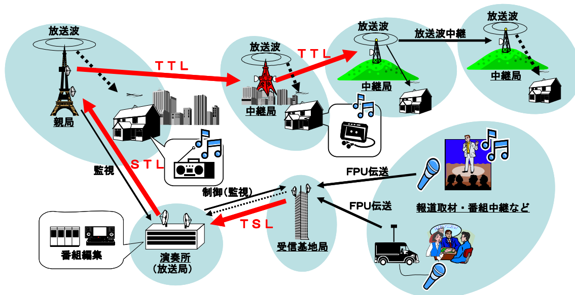
図1-1 音声STL/TTL/TSLの例
