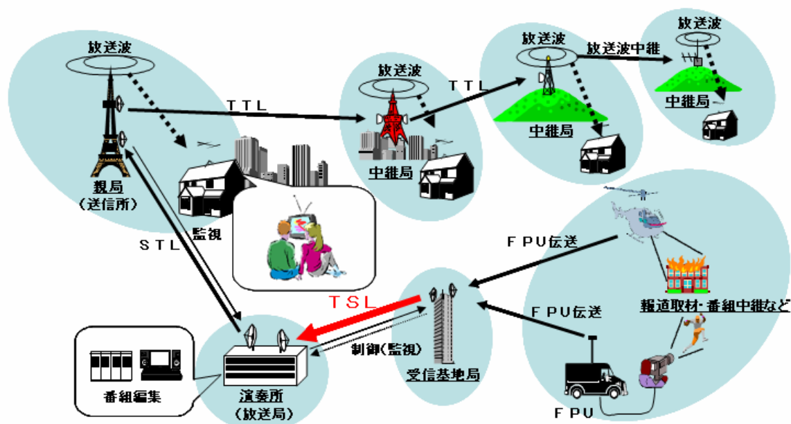
図 1-3 監視・制御用固定回線の例
