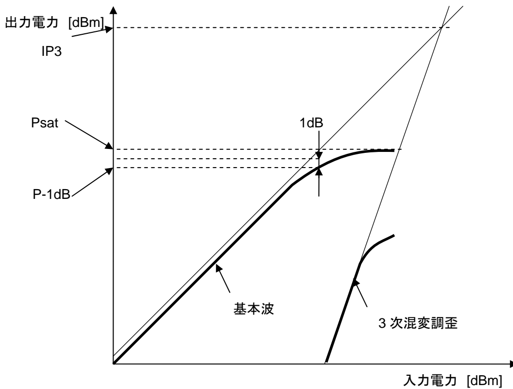
図1 P-1dB, Psat, IP3 の関係
