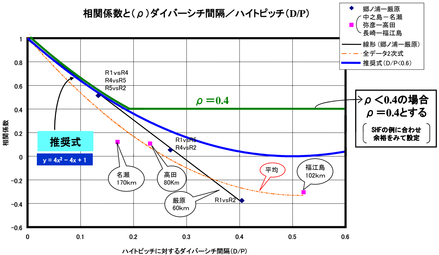
図1 ハイトピッチに対するダイバーシティ受信点位置と相関係数
