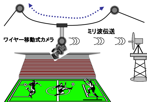
図 3-2 移動式(ワイヤー移動式)カメラにおけるミリ波伝送の運用例
