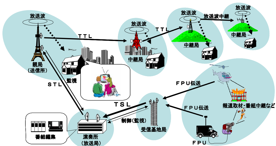
図1 テレビジョン放送ネットワーク例
