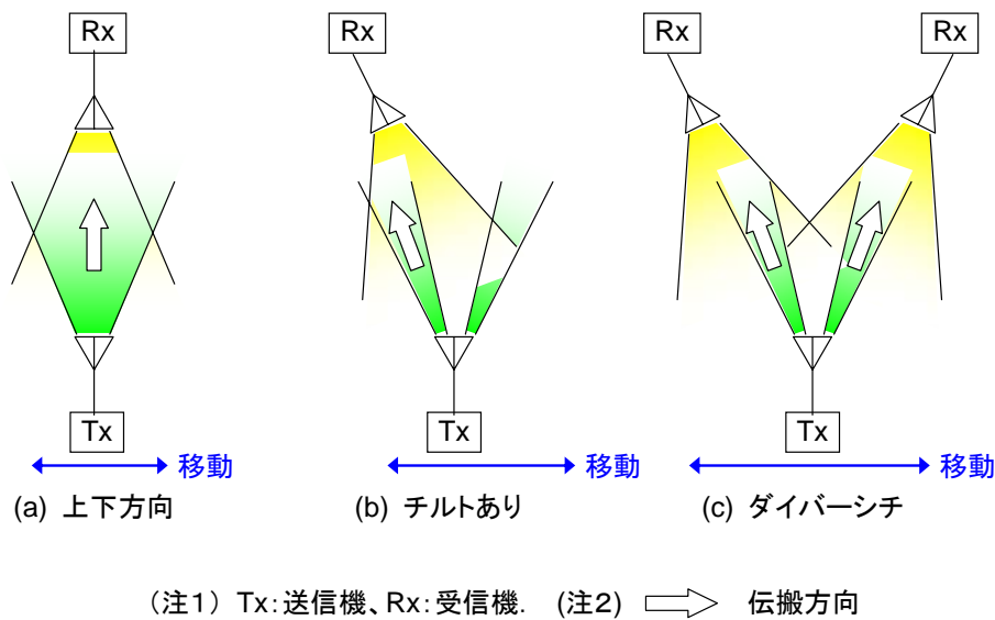
図1 スタジオ(天井が高い場合)で使用する送受信空中線の指向特性例
