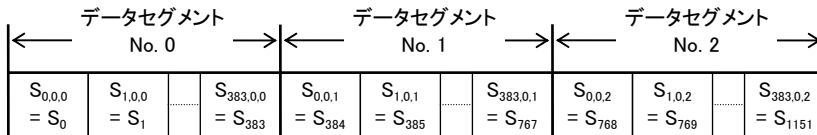
インターリーブ前のシンボル配置
