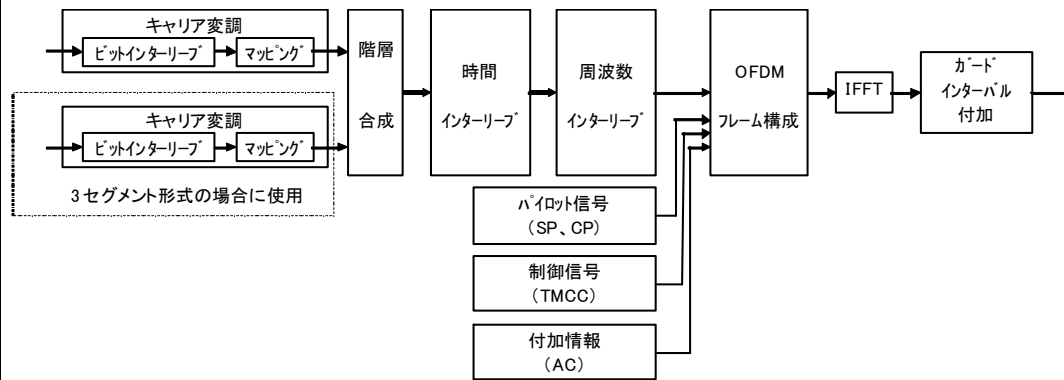
伝送路符号化部系統
