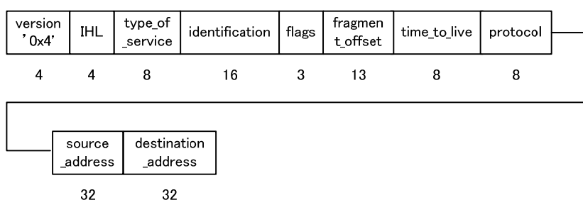
図3.4.3.2.1-2 IPv4_header_wo_length()の構成
