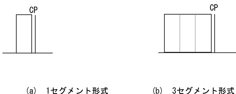
図3.6.2-1 単独送信のCPキャリア配置
