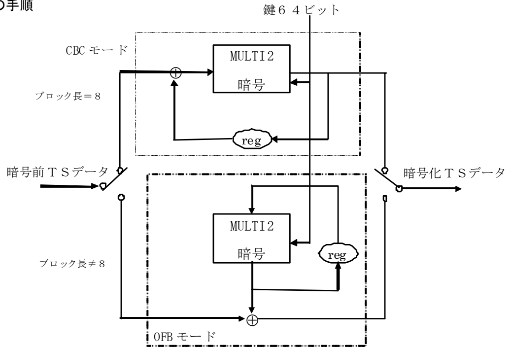
図 3.3.1-1 スクランブル方式
