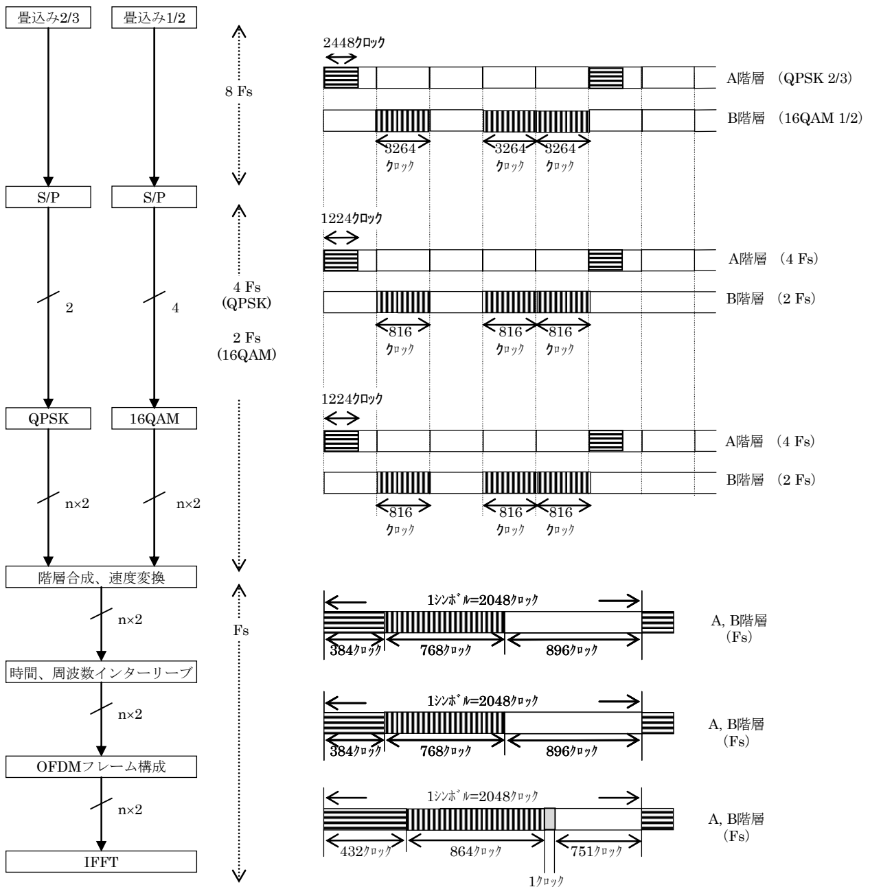
図3.5.16-1(b) 送信信号系統の例
