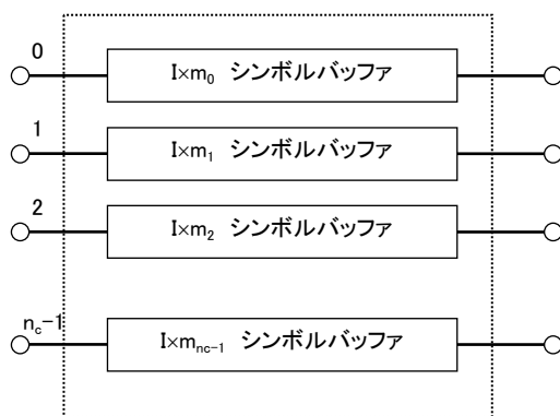
図3.5.11-2 セグメント内時間インターリーブの構成(告示第四十一号 別表第二号 別記第2)
