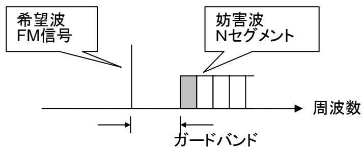
図5-2 希望波と妨害波の配置図
