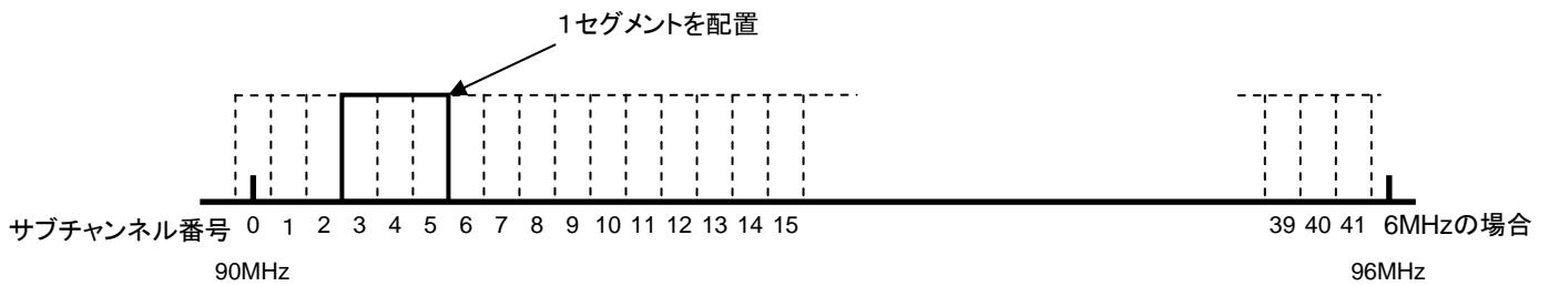
図5.3-1 サブチャンネル番号の定義
