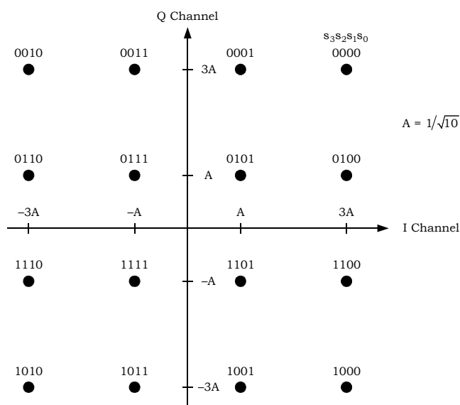
図3.5.15.2-1. 16QAM位相図
