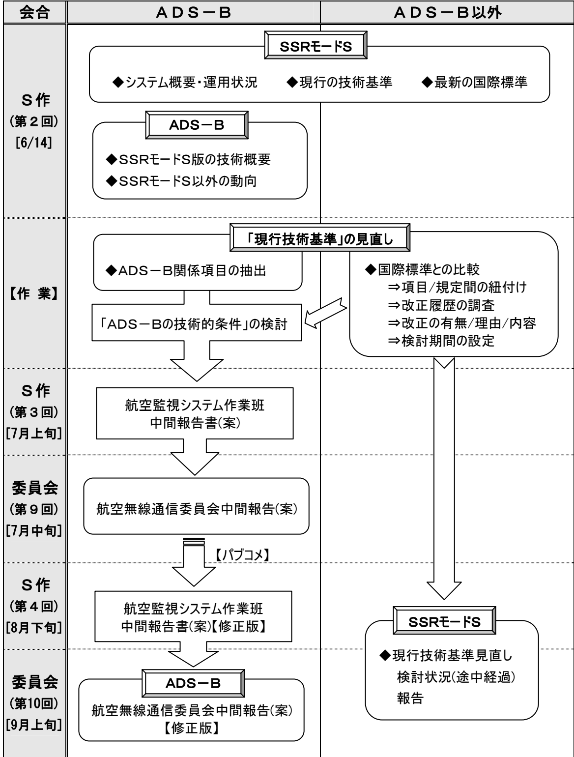
【参考】流れ図
