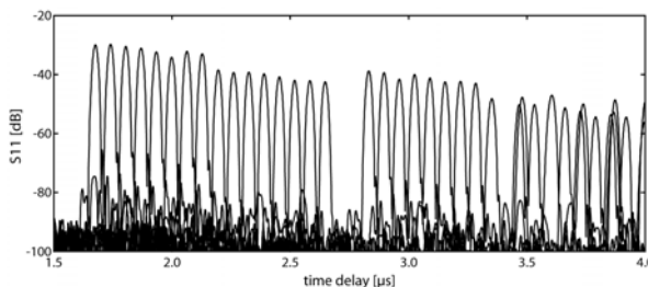
試作 SAW センサの動作例
