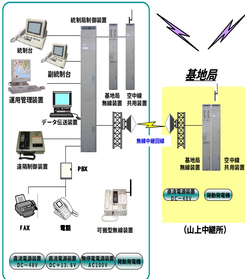
【市町村デジタル移動通信システムの構成】
