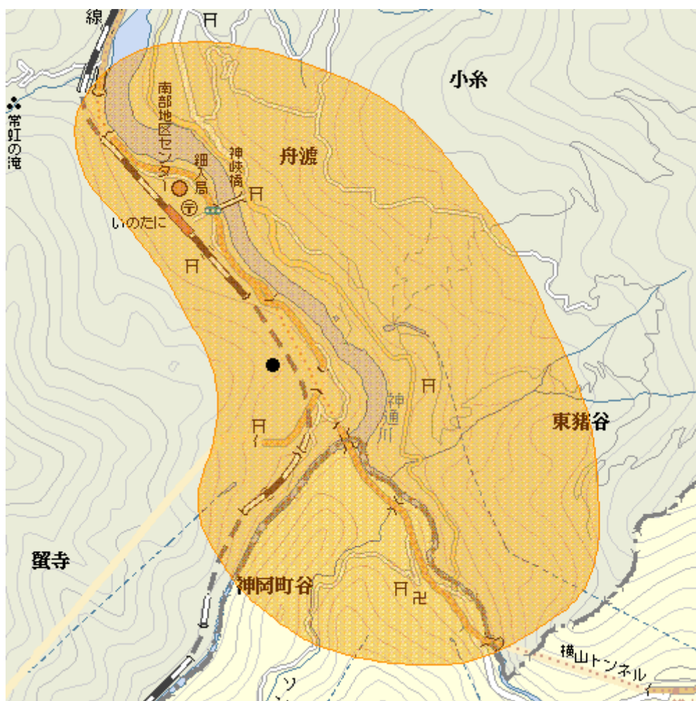
<細入猪谷中継局エリア図>
