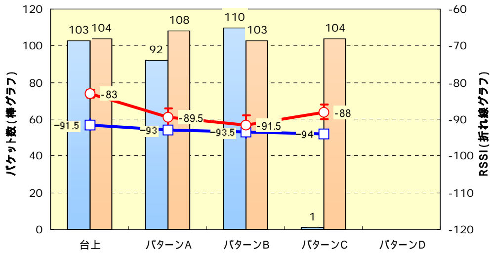
図 12 30m パターン特性
