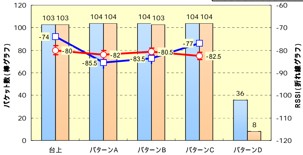
図 10 10m パターン特性
