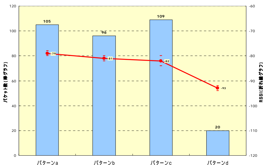
図 17 親機 135cm、10m パターン特性 (向き)
