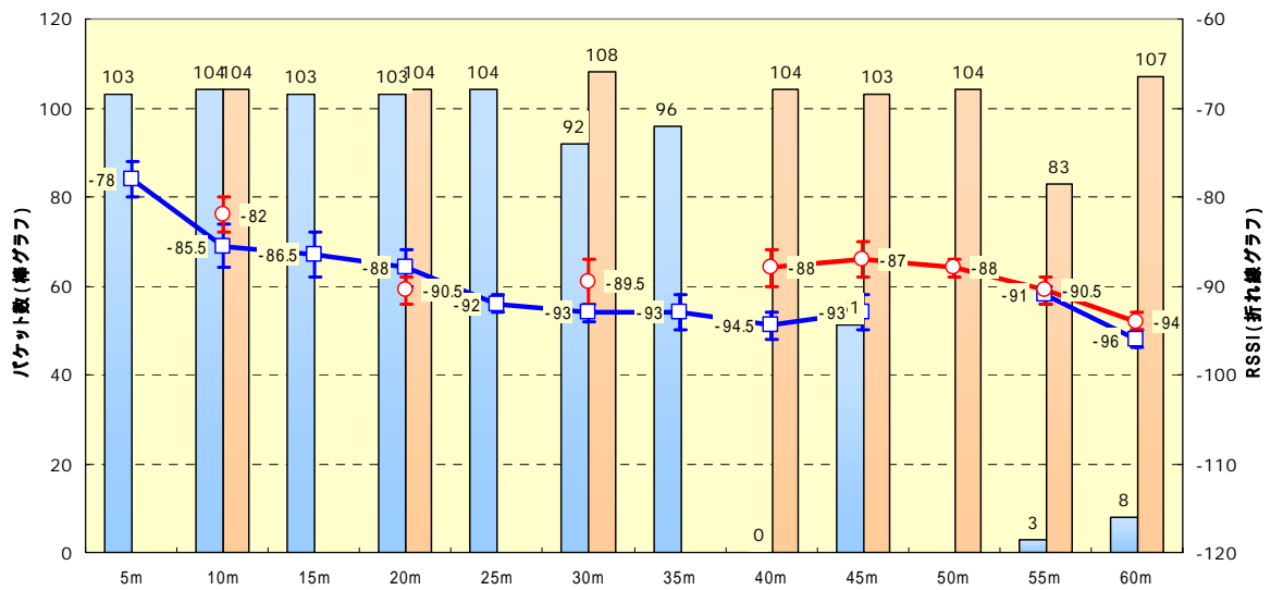
図6 パターン A 距離特性
