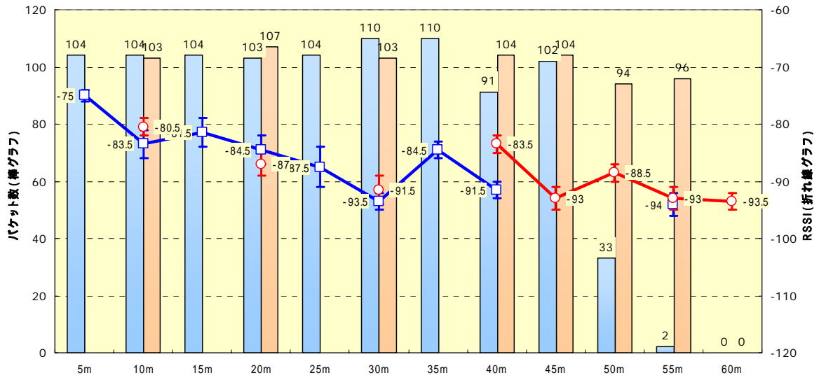
図7 パターンB 距離特性
