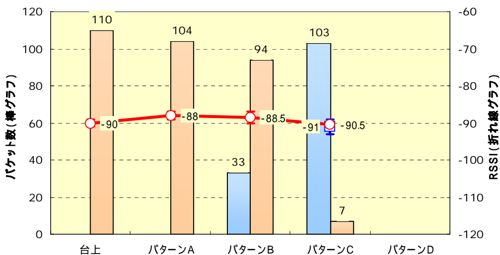
図 14 50m パターン特性
