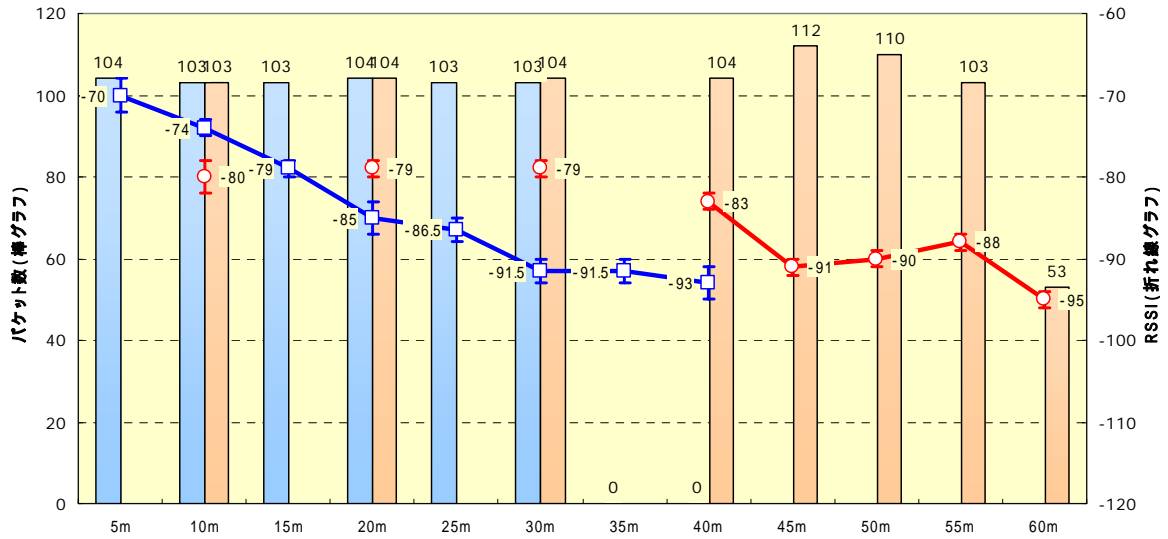
図5 台上パターン距離特性
