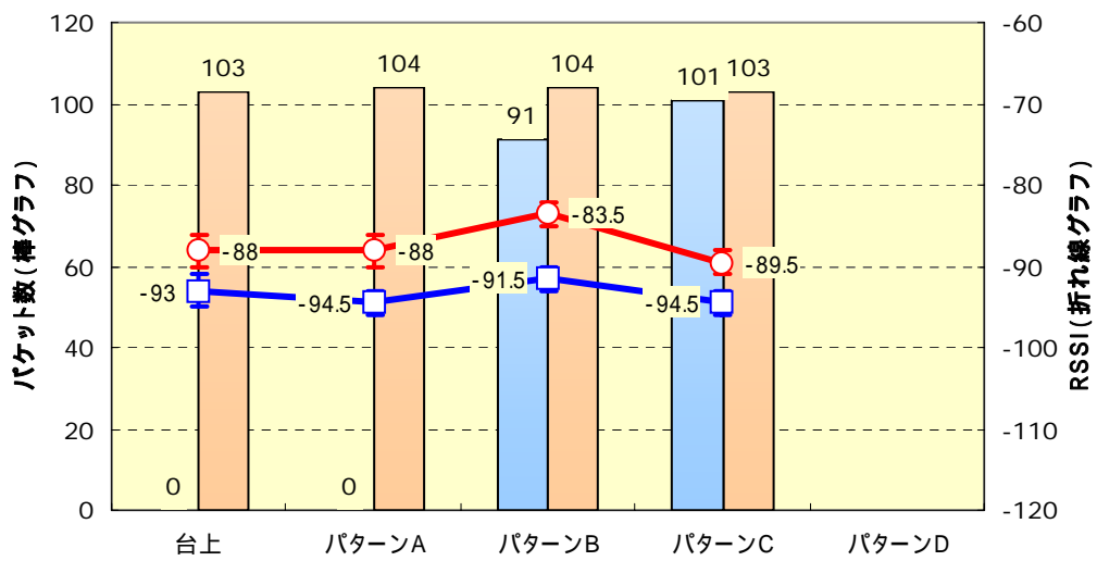
図 13 40m パターン特性
