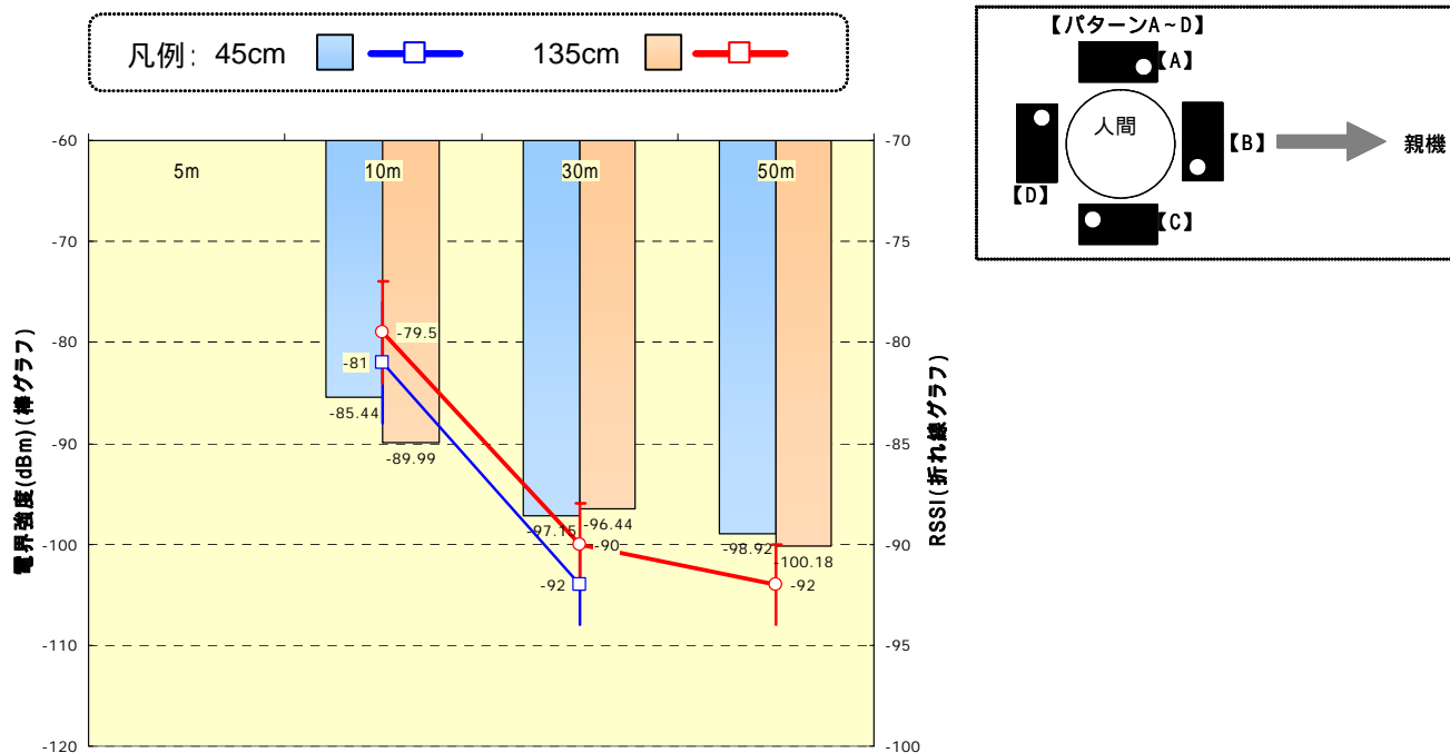
図 2 台上 RSSI・電界強度特性
