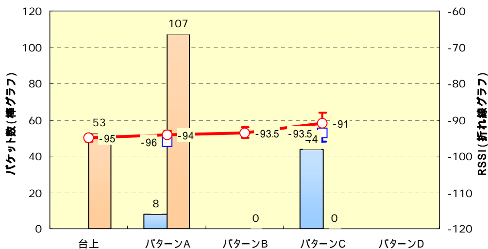
図 15 60m パターン特性
