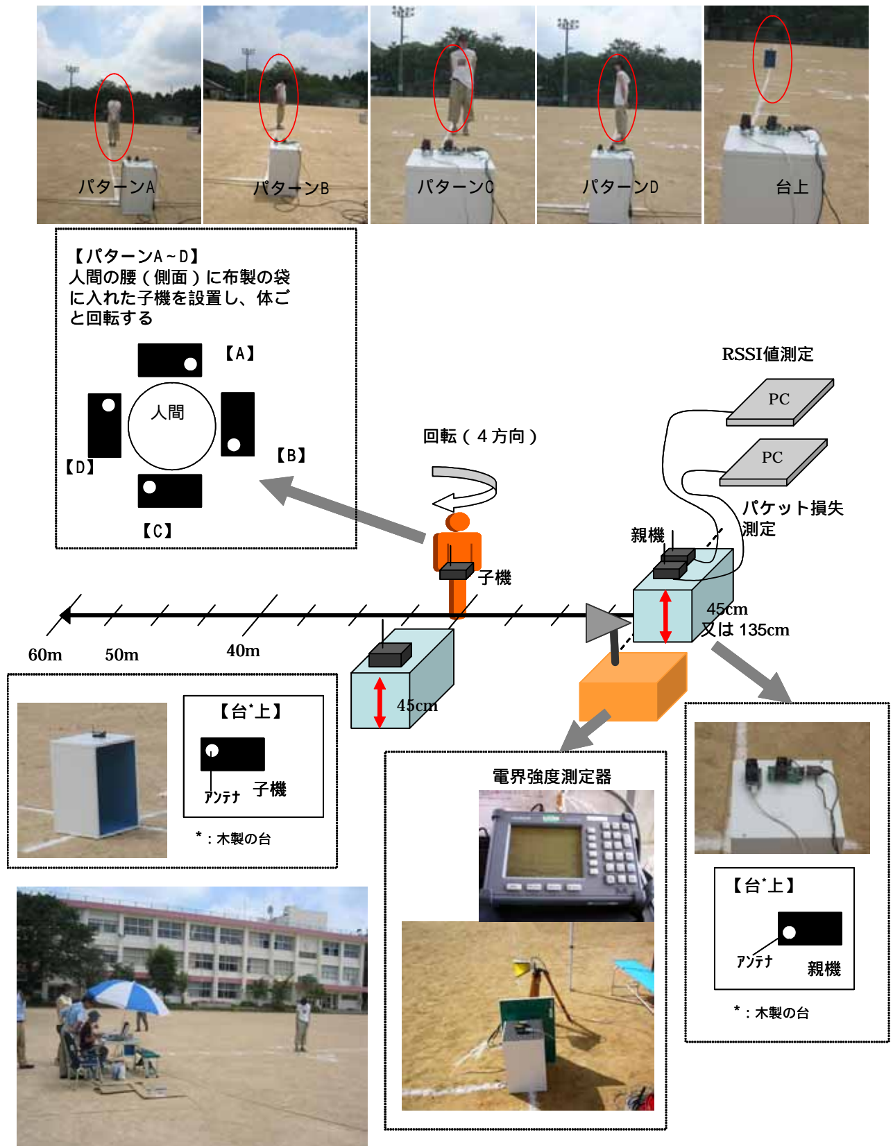
図1 電波伝搬特性試験イメージ
