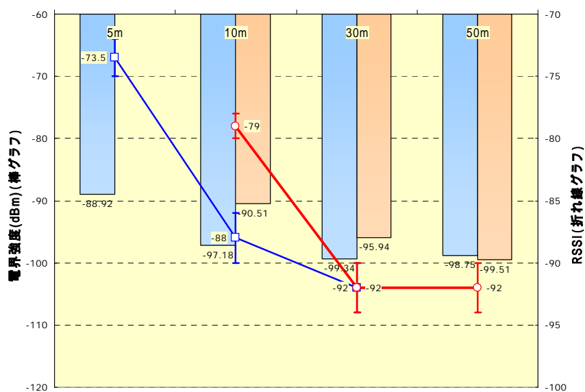
図 3 パターン B RSSI・電界強度特性
