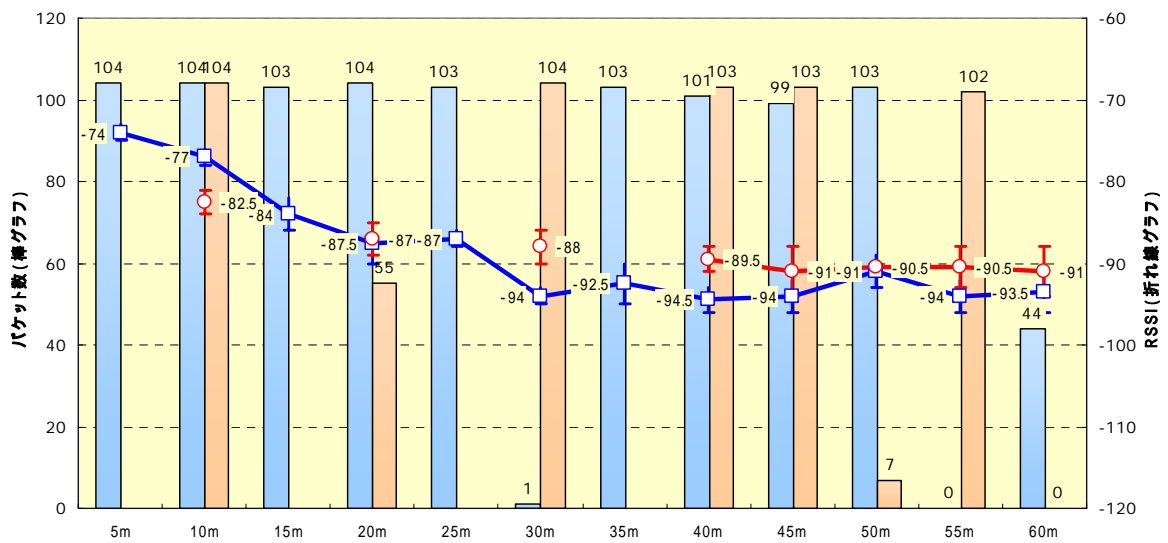
図8 パターンC 距離特性
