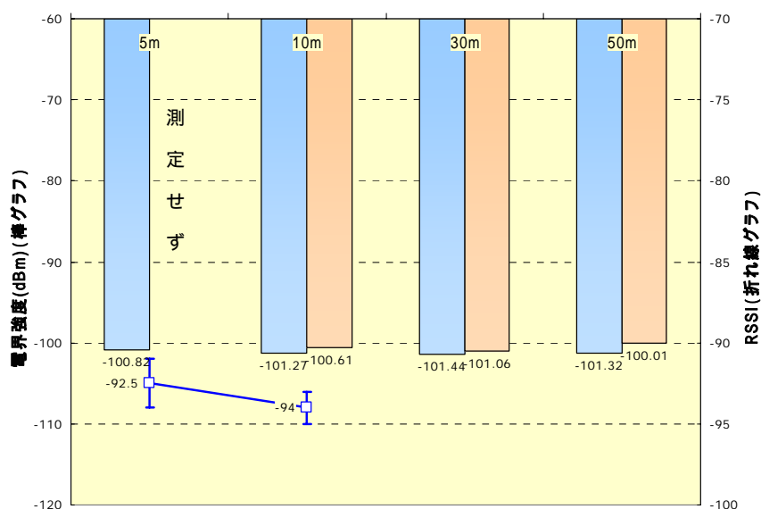
図4 パターンD RSSI・電界強度特性
