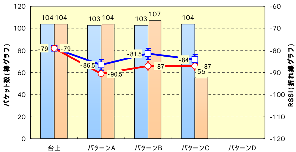
図 11 20m パターン特性
