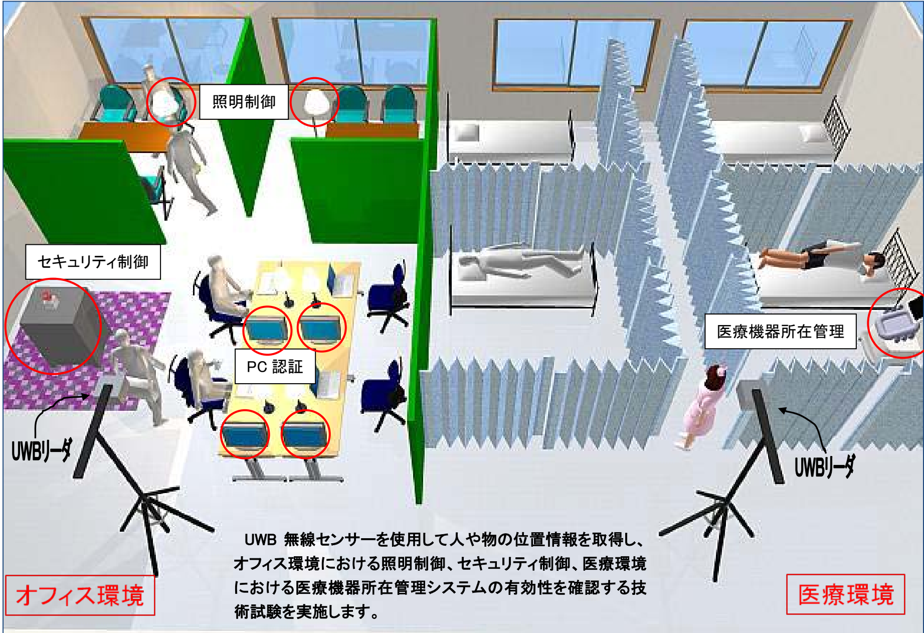
オフィス並びに医療環境を擬似的に構築した利用モデルシステムの全景イメージ
