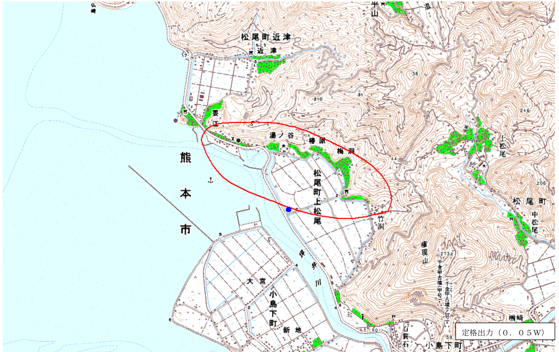
松尾西中継局放送区域図
