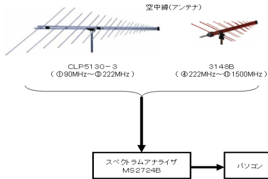
測定系の構成
